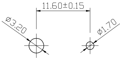
P.C.B. LAYOUT (印刷电路板配置)
