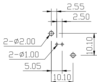
(1 : 1) P.C.B. LAYOUT (印刷电路板配置)
