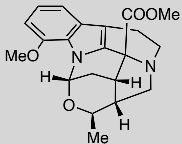
(+)-Alstroline G
