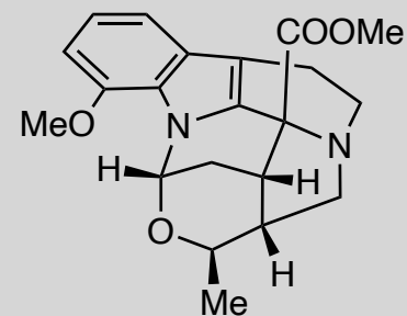
(+)-Alstroline G
