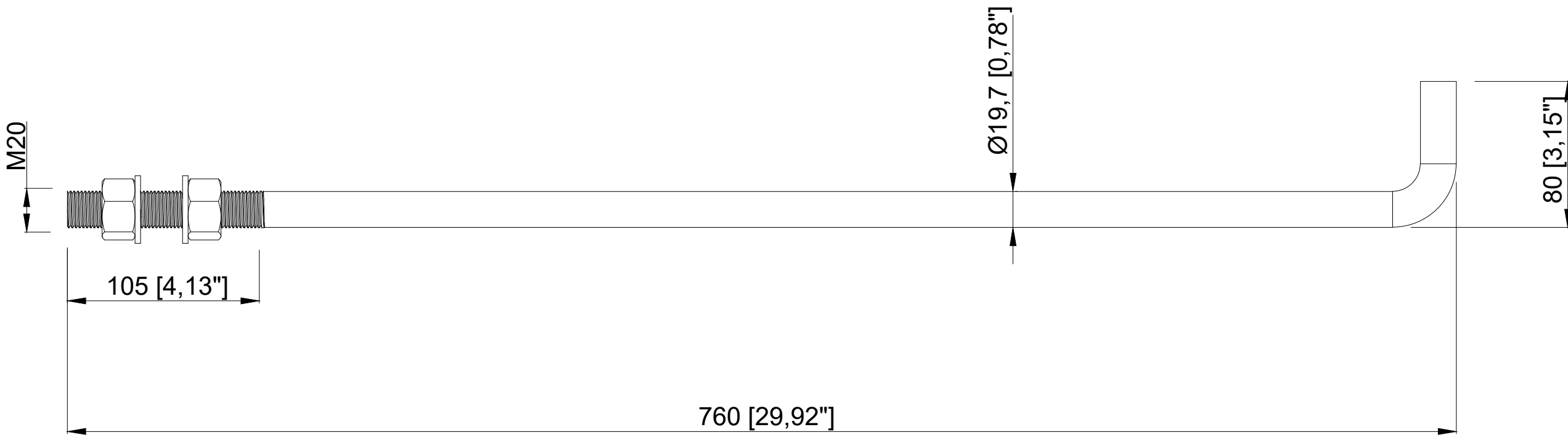
ANCHOR BOLT 4PCS PER POLE
