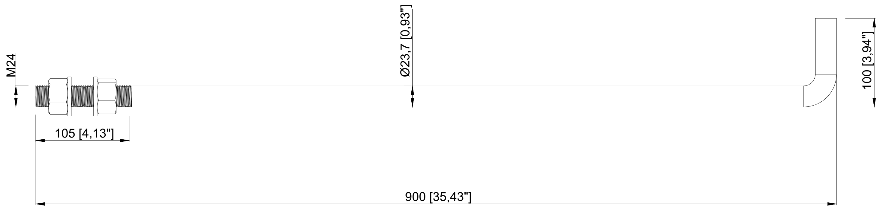
ANCHOR BOLT 4PCS PER POLE
