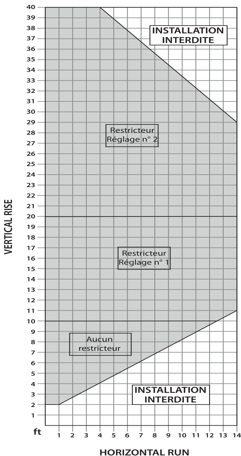
Figure 24: Configurations d'évent pour terminaisons verticale possible et terminaisons horizontale.
