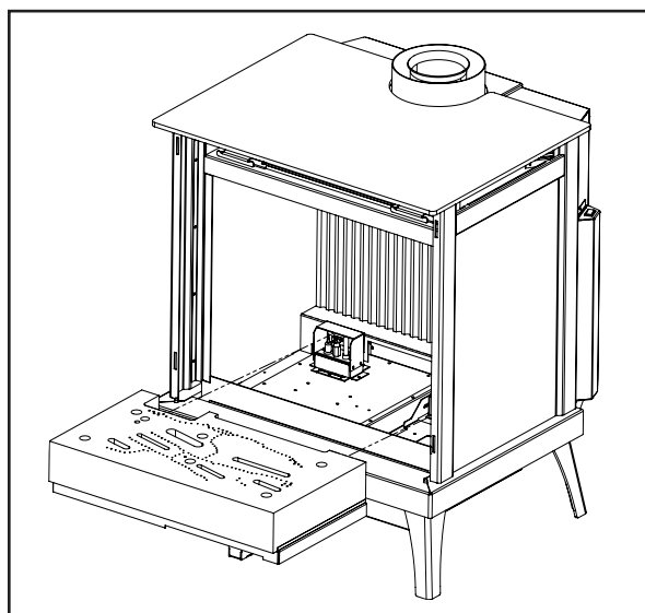
Figure 11. Enlever le brûleur
