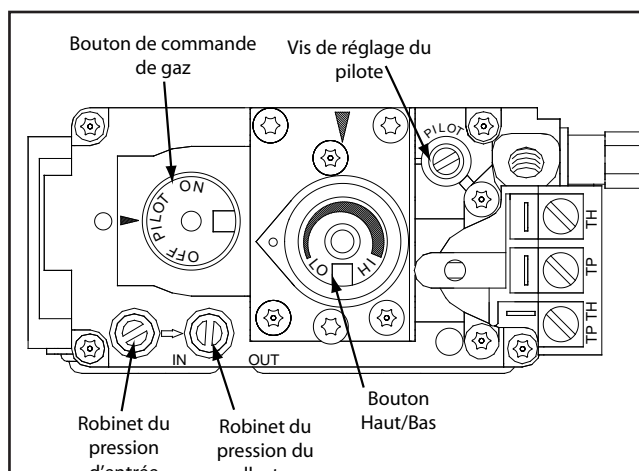
Figure 36: Robinet de gaz entièrement étiquetée.
