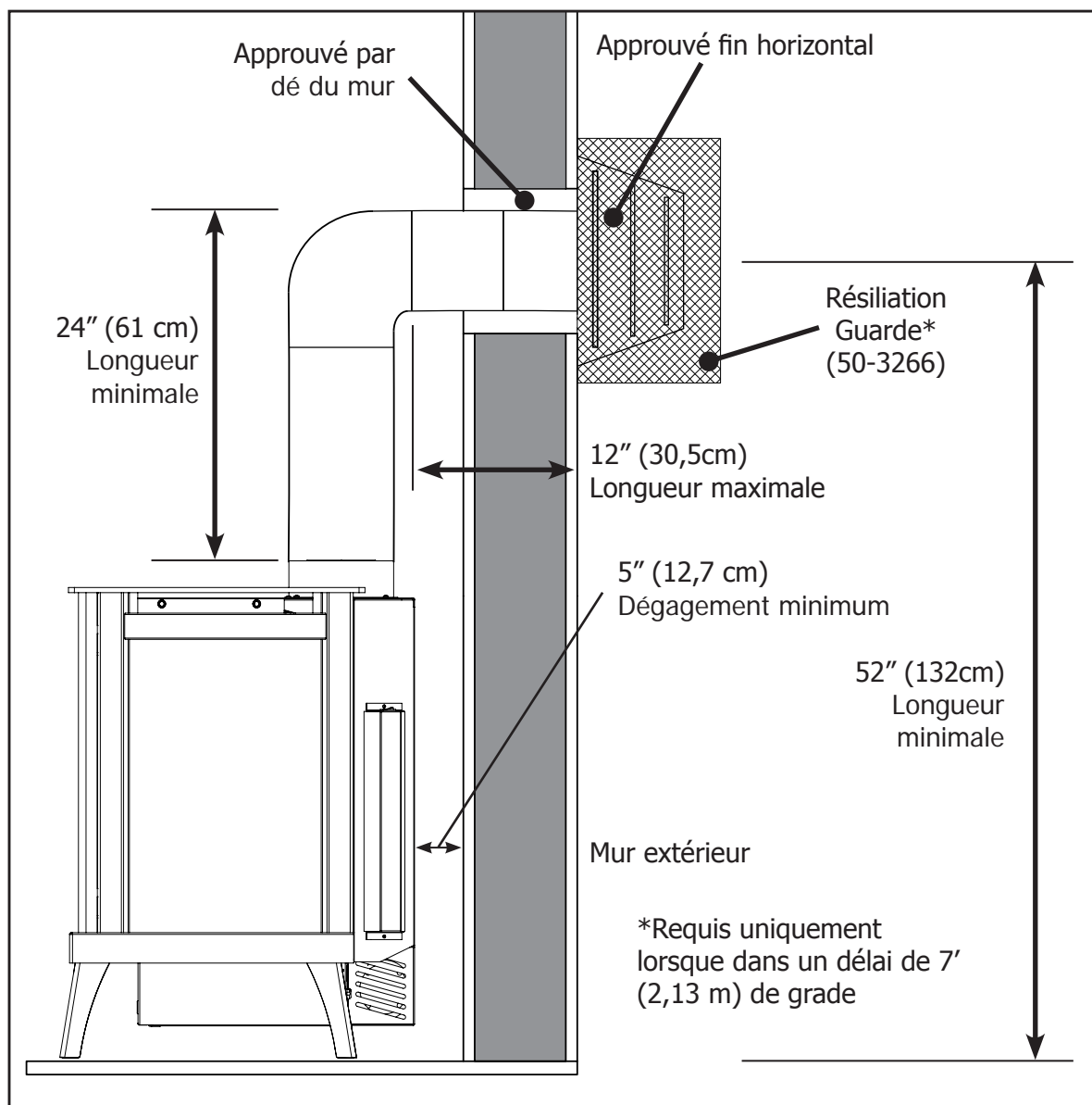
Figure 22. Longueur minimale d'évent
