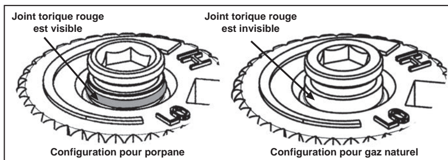
Figure 17: L'anneau de la vis de la vanne.
