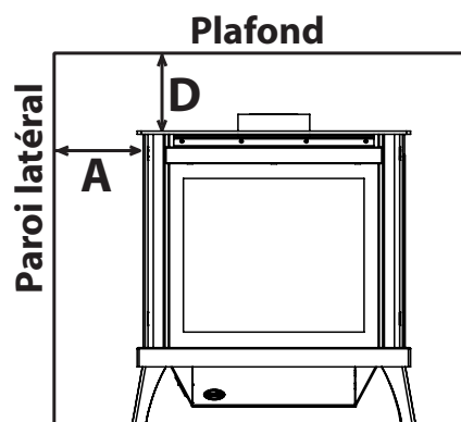
Figure 20 : Distance aux Combustibles
