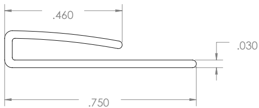
Edge Trim
