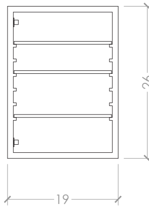
BOX DIMENSIONS
