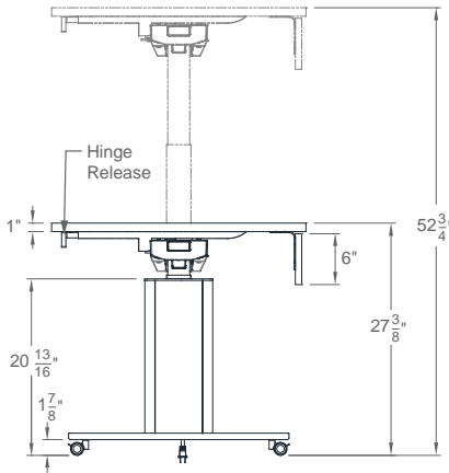
END ELEVATION
