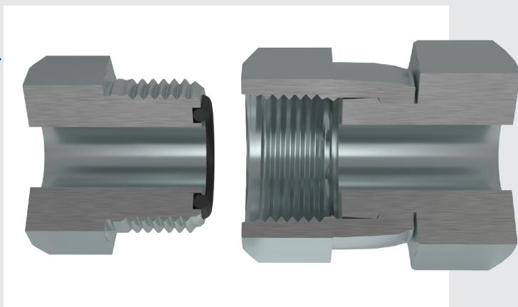
SAE (ORFS)
