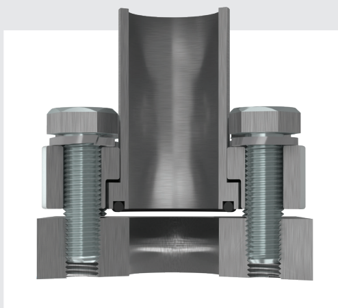
JIS 4-Bolt Flange
