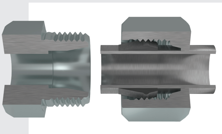
DIN EN ISO 8434-1 Standard
