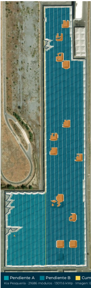
Fila 1 continua // borde largo (rumbo 0°). Setback 5 m (línea teal). Gable ~4° az 270°/90°. Portrait, largo // costuras (S-5!). No sustituye visita técnica.
