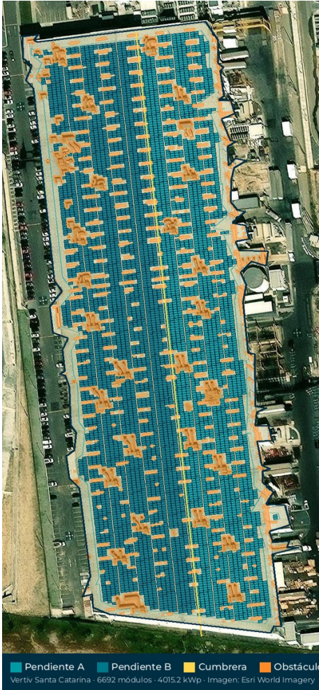
Fila 1 continua // borde largo (rumbo 174°). Setback 5 m (línea teal). Gable ~4° az 84°/264°. Portrait, largo // costuras (S-S!). No sustituye visita técnica.
