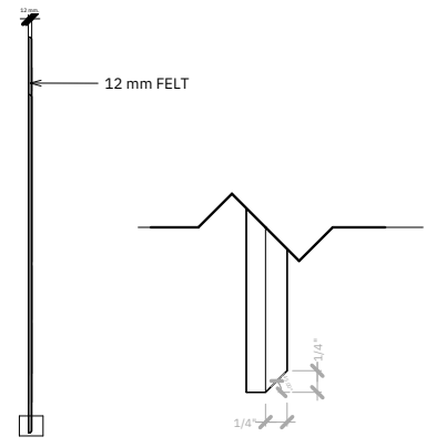
3 EDGE DETAIL
