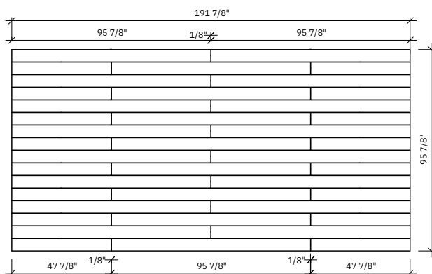
2 AOUDI DIMENSIONS - FACE
