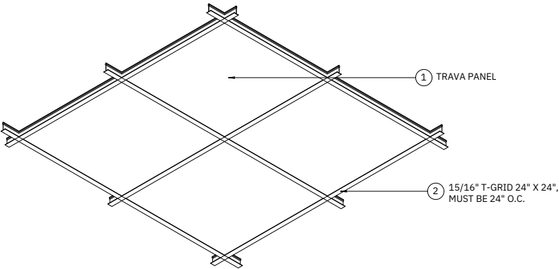
2 TRAVA - LAY IN - BOTTOM DIMETRIC
