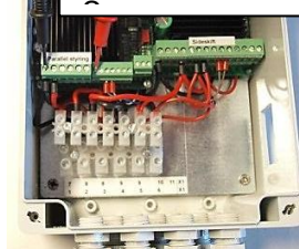
Actuator 2, aansluitpolen 1 en 11 + 1
