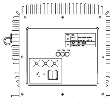
Figuur 2-23. Acculader
