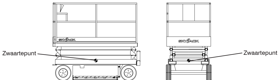
Figuur 2-18. Zwaartepunt
