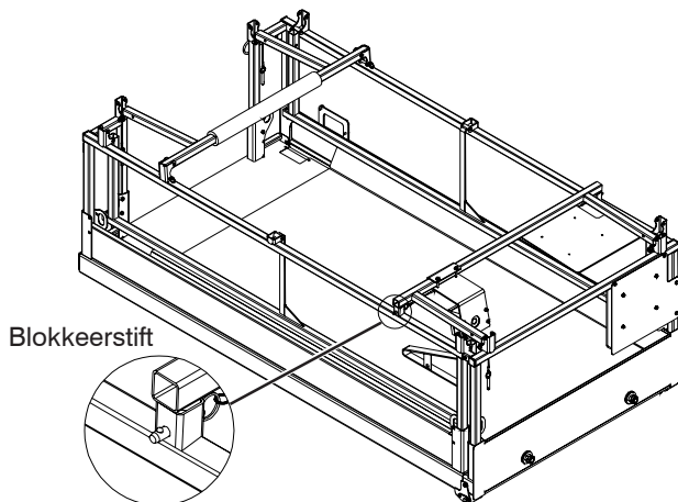
Figuur 2-12b. Alle relingen toegevouwen
