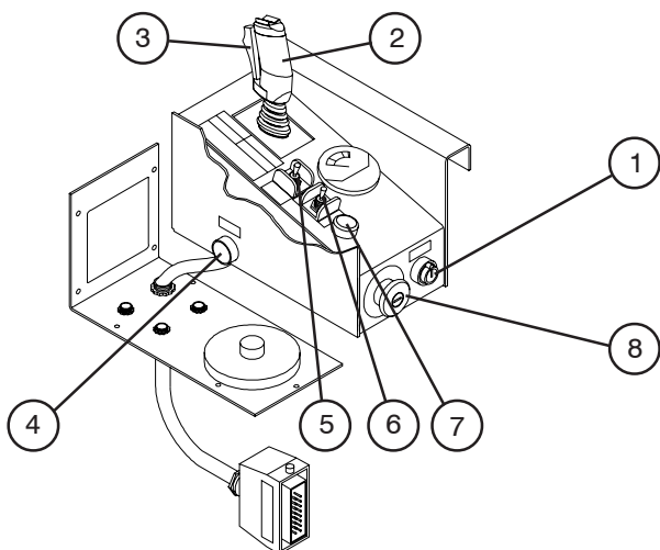
Figuur 2-10. Bedieningspaneel
