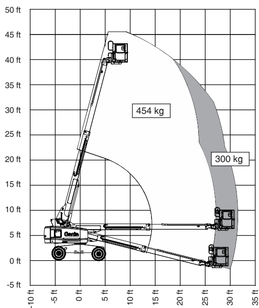
Diagram werkbereik S-40 XC en S-40 TRAX
