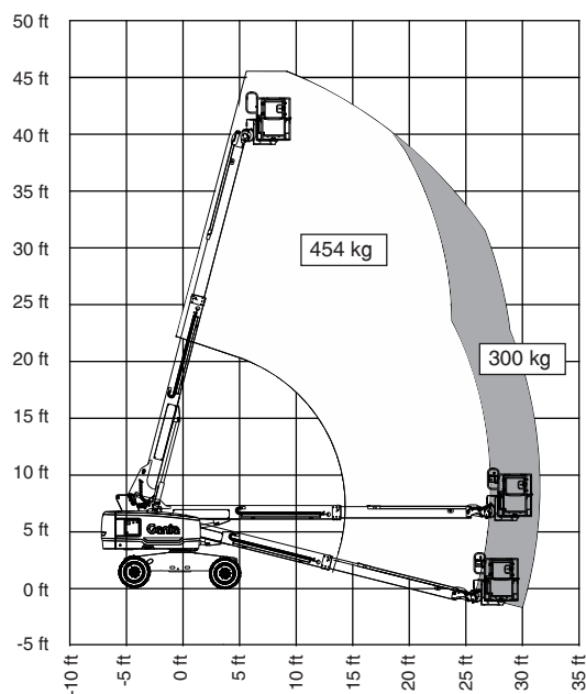
Diagram werkbereik S-45 XC en S-45 TRAX
