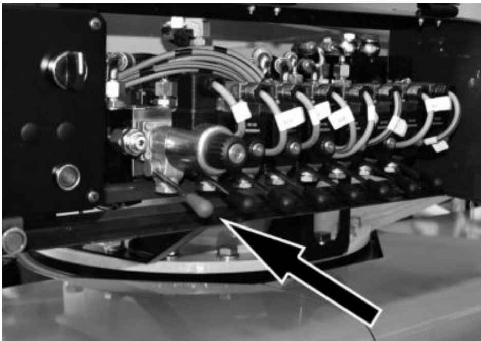
Fig. 75 Knop activering proportionele klep hoogwerkerdeel
