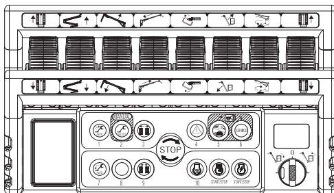
Fig. 107 Afstandsbediening
