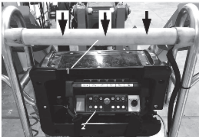
Fig. 60 1-Sensor SkyGuard™ 2- SkyGuard™ By-pass (knop nummer 8)
