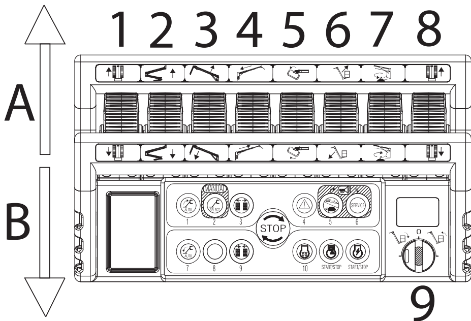
Fig. 50 Bedieningen joysticks
