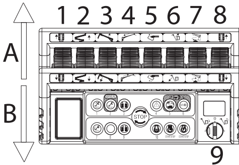
Fig. 109 Bedieningen joysticks
