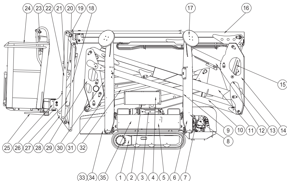
Fig. 6 Begrippen componenten machine
