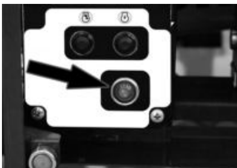
Fig. 114 Verklapper toestemming hoogwerkerdeel noodbedieningspaneel
