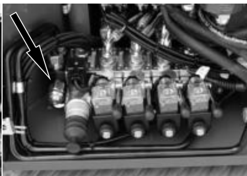
Fig. 10 Overdrukklep wagen
