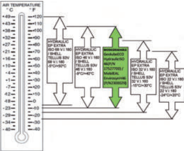
Fig. 150 Gebruikstemperaturen olie
