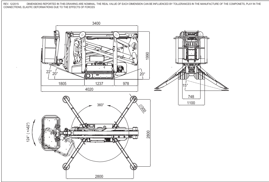
Fig. 5 Standaardversie met tweepersoonsbak
