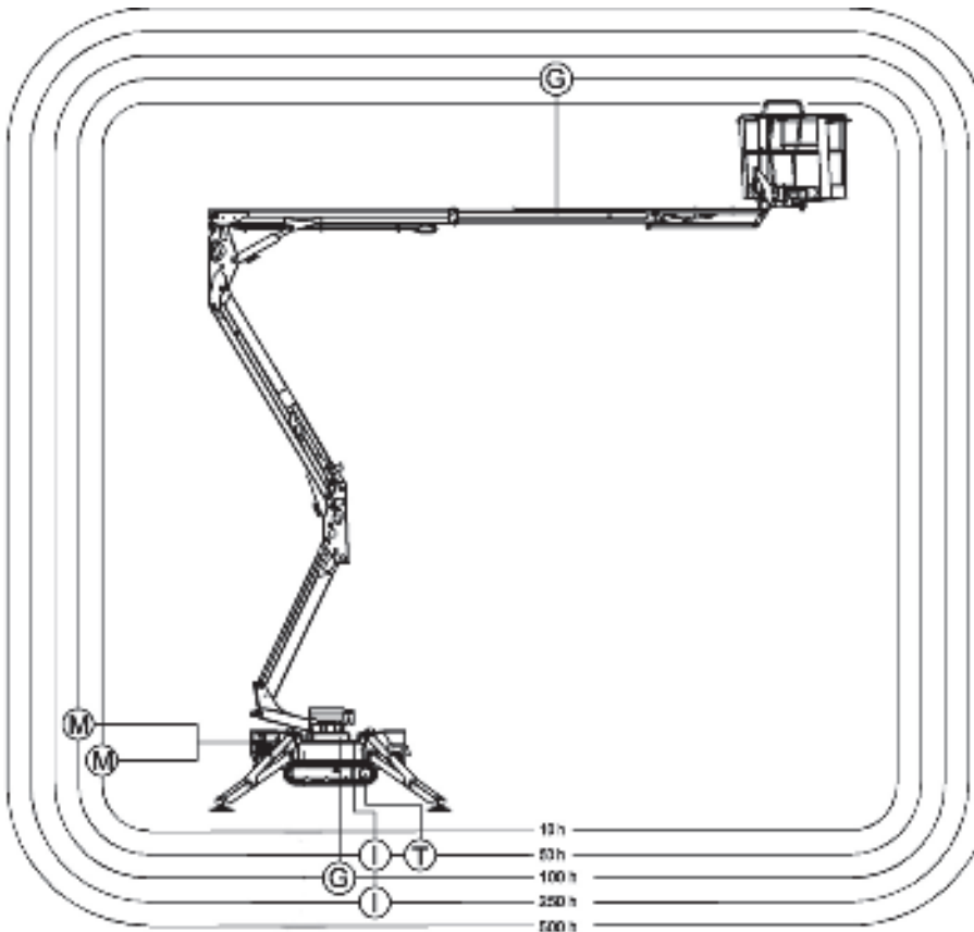
Fig. 152 Schema Smeerpunten
