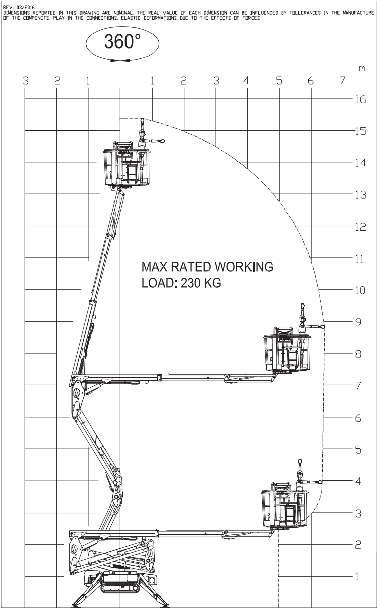
Fig. 80 Werkzone
