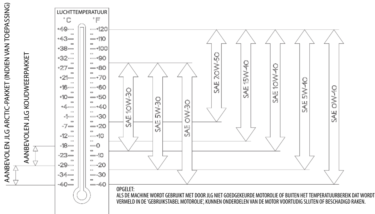
Figuur 7-2. Specificaties motorbedrijfstemperatuur – Deutz
