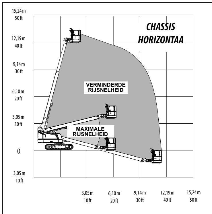
Figuur 4-5. Schema's werkbereik rijfunctie - Blad 1 van 2
