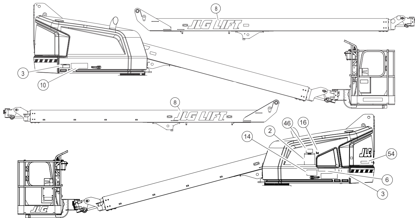
Figuur 4-9. Plaats van stickers – Draaischijf – Blad 1 van 3
