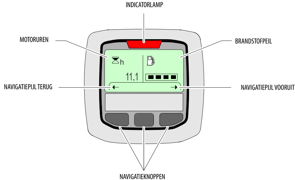
Figuur 3-7. Weergavemeter grondbedieningsconsole
