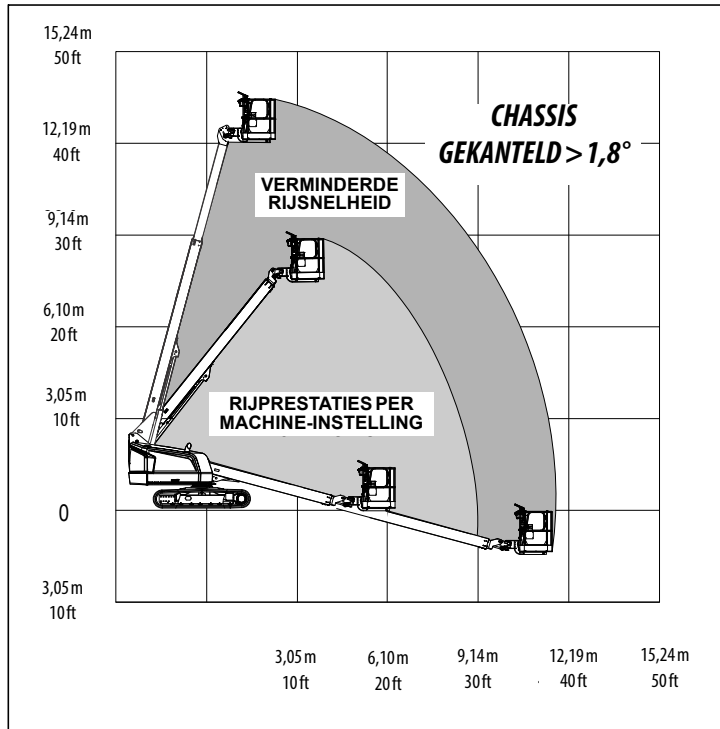
Figuur 4-6. Schema's werkbereik rijfunctie - Blad 2 van 2
