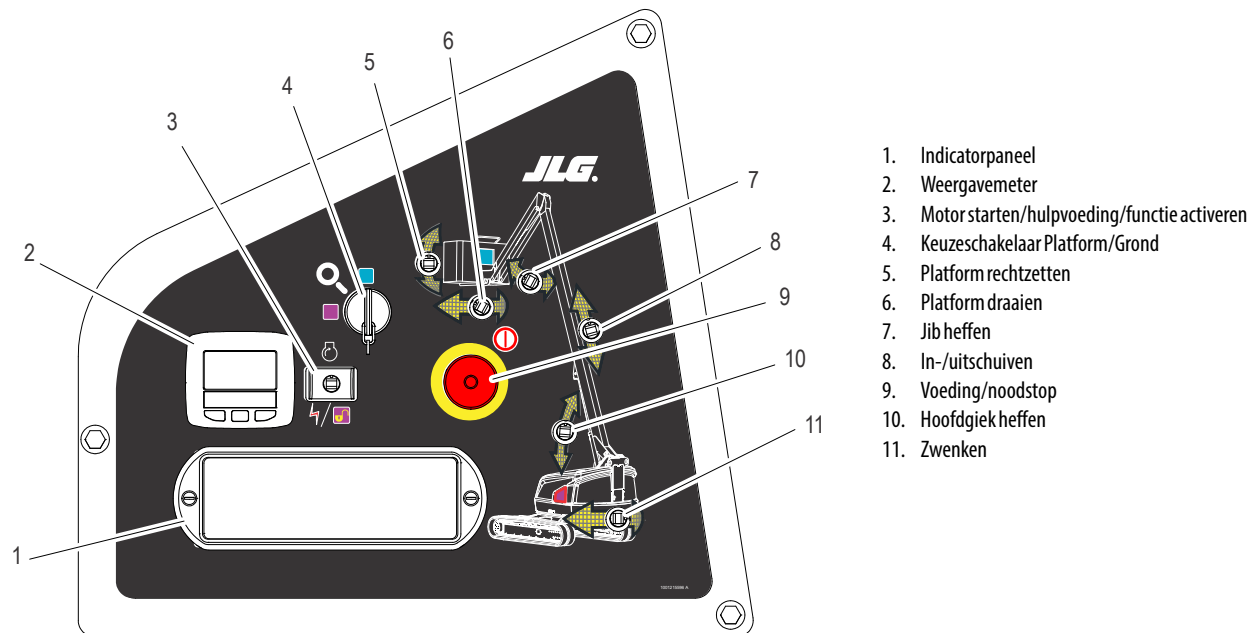
Figuur 3-2. Grondbedieningsconsole – 460SJC
