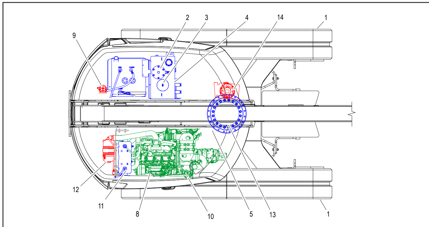
Figuur 7-6. Schema voor smering en onderhoud door machinist – Deutz 2,9 L4
