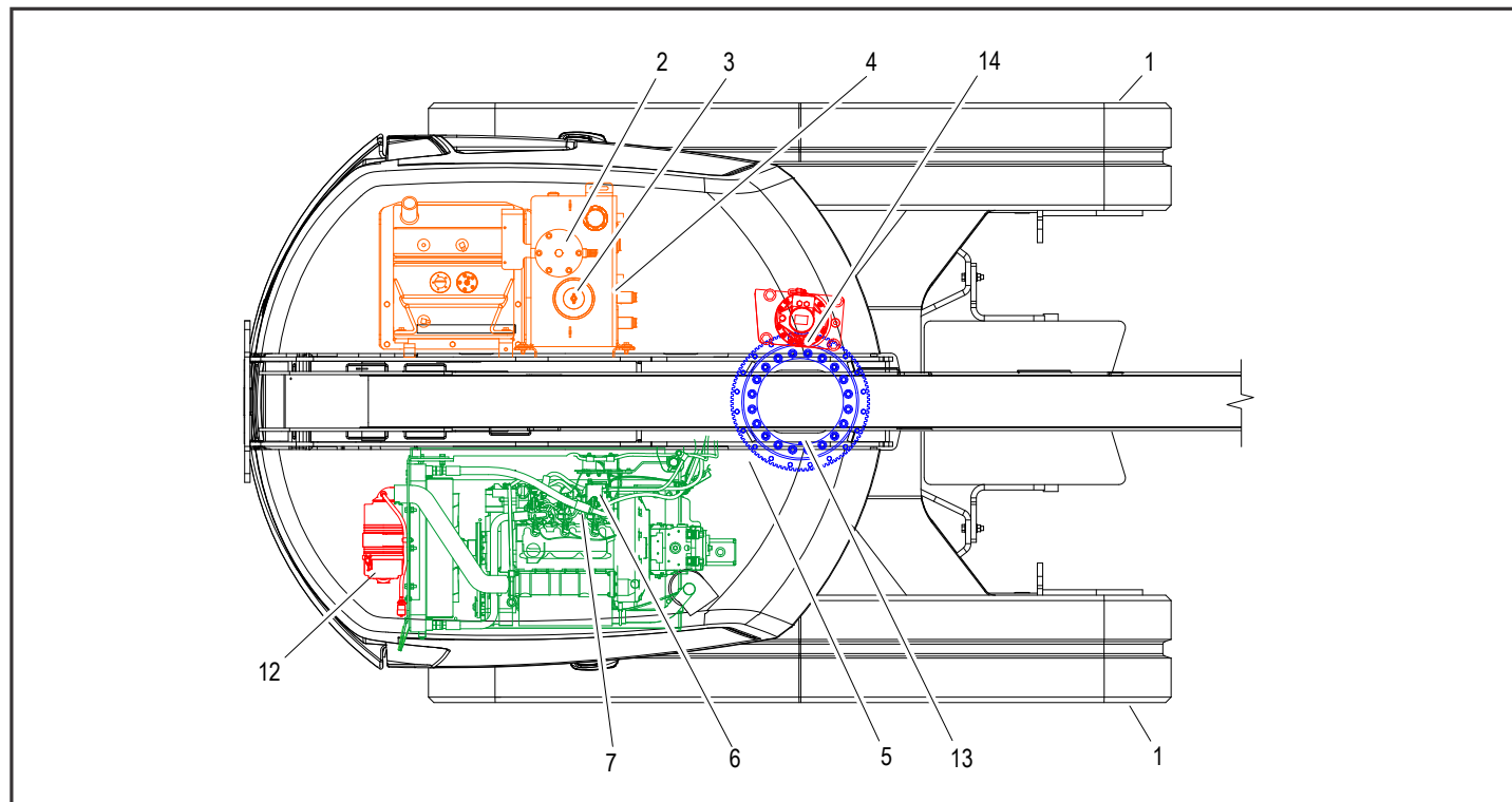
Figuur 7-5. Schema voor smering en onderhoud door machinist – Deutz D2011
