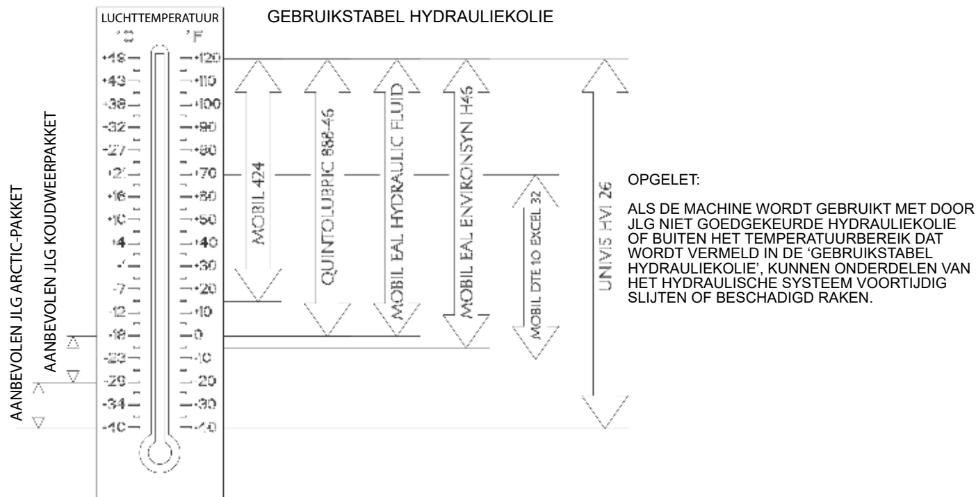
Figuur 7-3. Gebruikstabel hydrauliekolie – Blad 1 van 2
