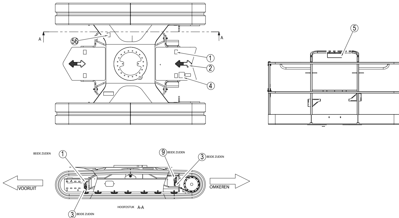
Figuur 4-12. Plaats van stickers – Chassis
