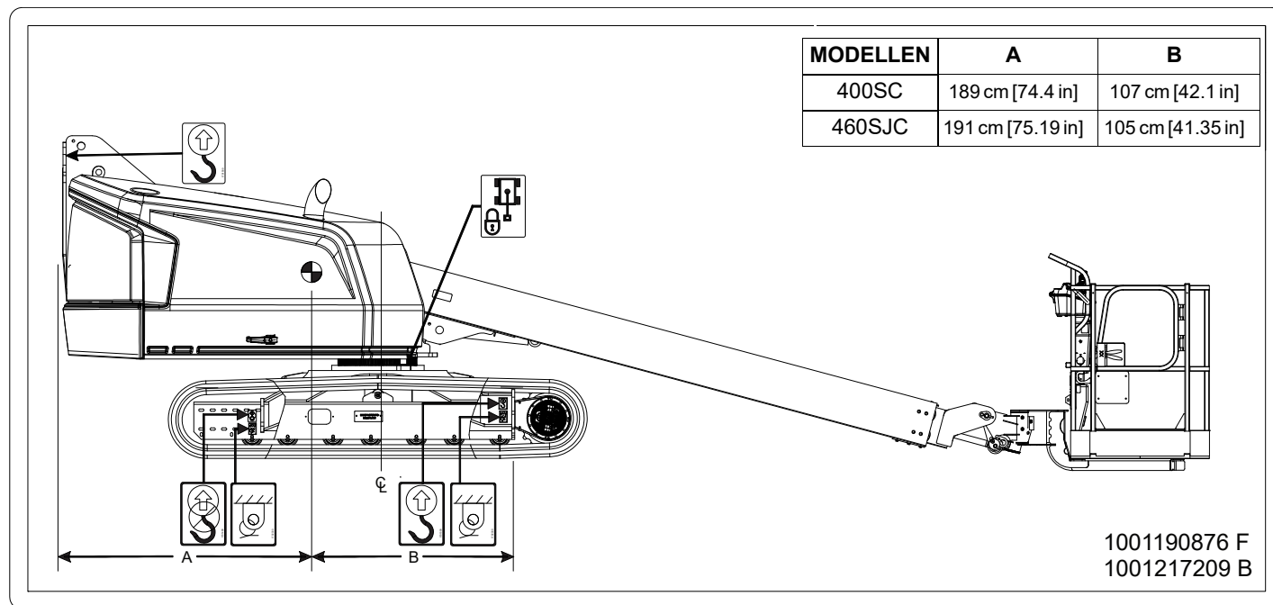
Figuur 4-8. Tabel voor hijsen en vastsjorren
