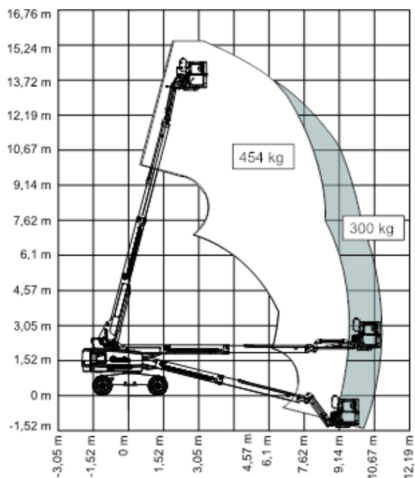
Diagram werkbereik S-45 XC en S-45 TRAX
