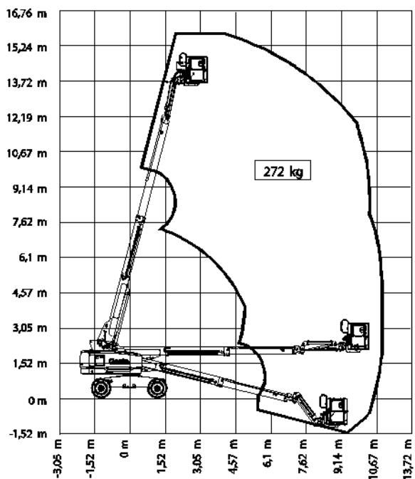
S-45 HF Diagram werkbereik
