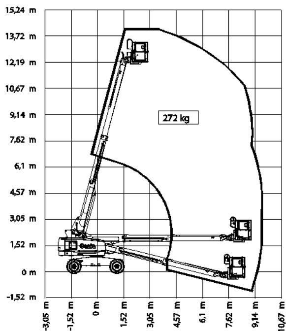
S-40 HF Diagram werkbereik
