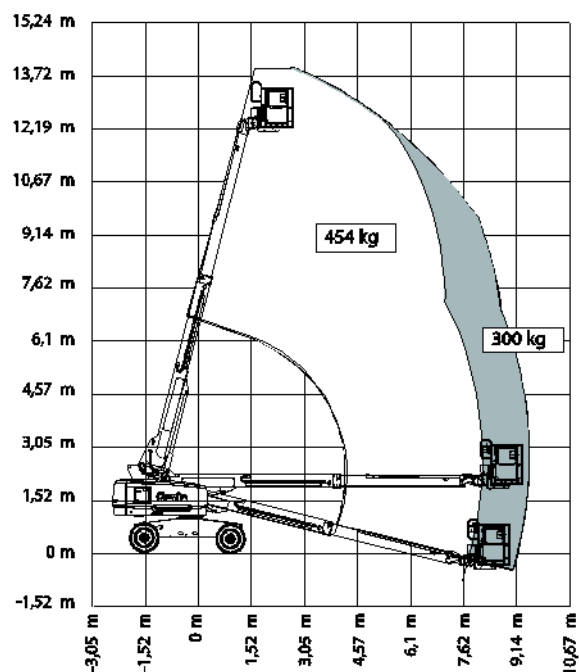
S-45 XC en S-45 TRAX Diagram werkbereik
