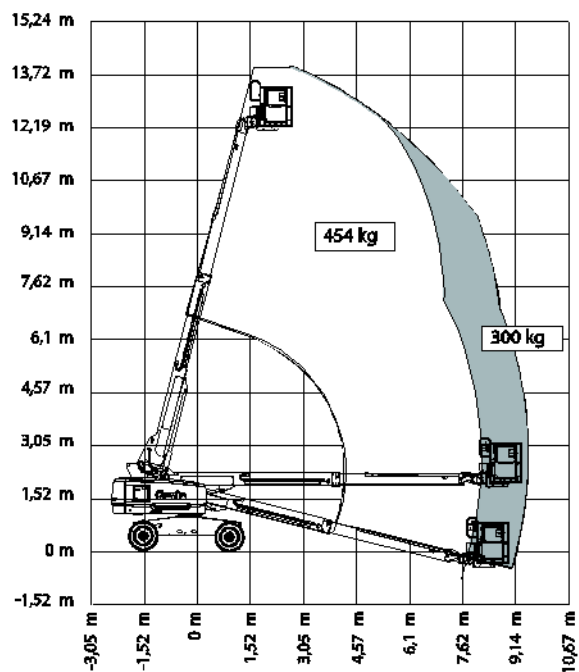
Diagram werkbereik S-40 XC en S-40 TRAX
