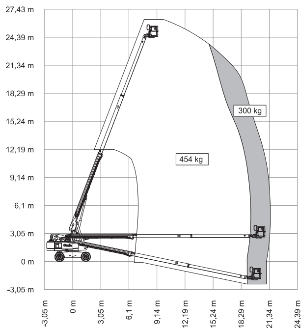
Diagram werkbereik S-80 XC
