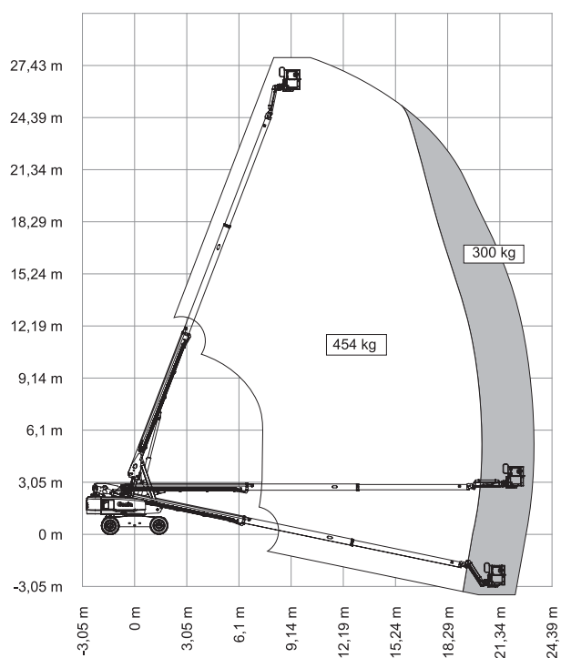
Diagram werkbereik S-85 XC
