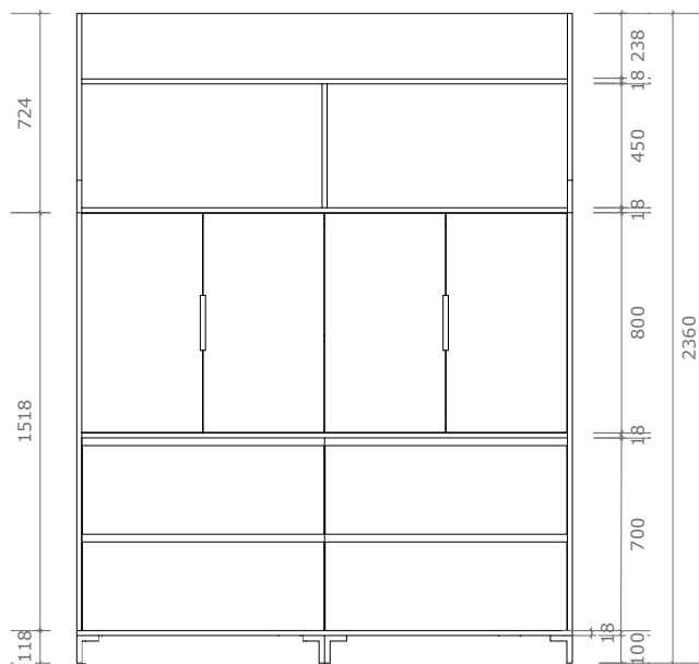
ALZADO 1 - Puertas cerradas
