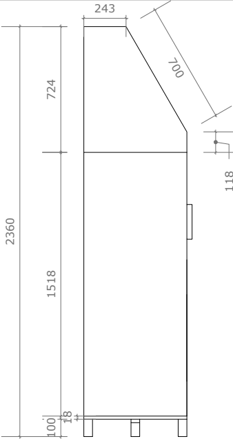
ALZADO 4 - Perfil
