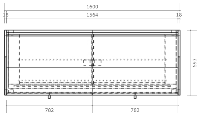
PLANTA
