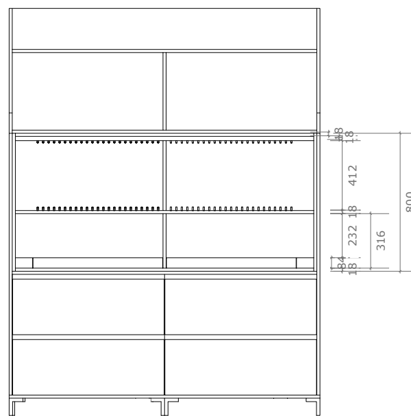
ALZADO 2 - Interior
