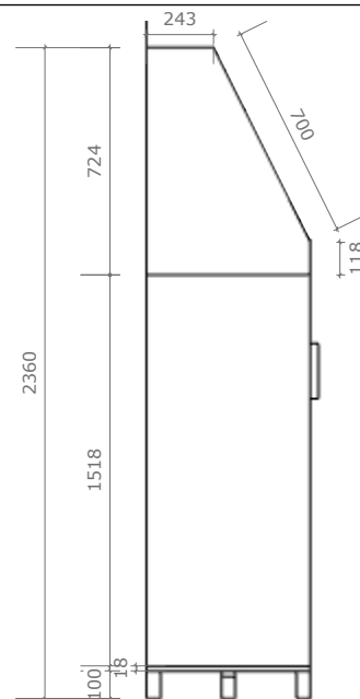
ALZADO 4 - Perfil
