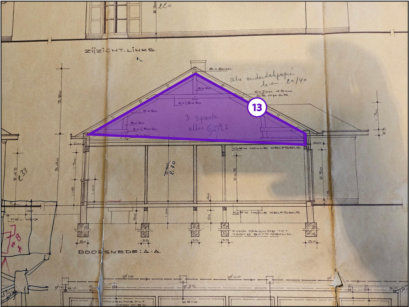
Legende van plan 1.9: Doorsnede
