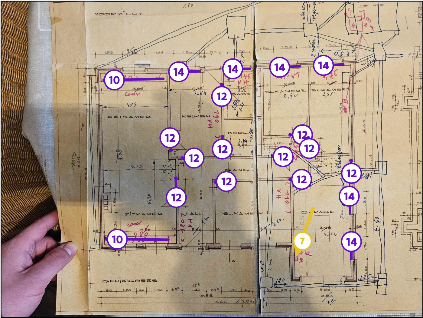
Legende van plan 1.3: Gelijkvloers
