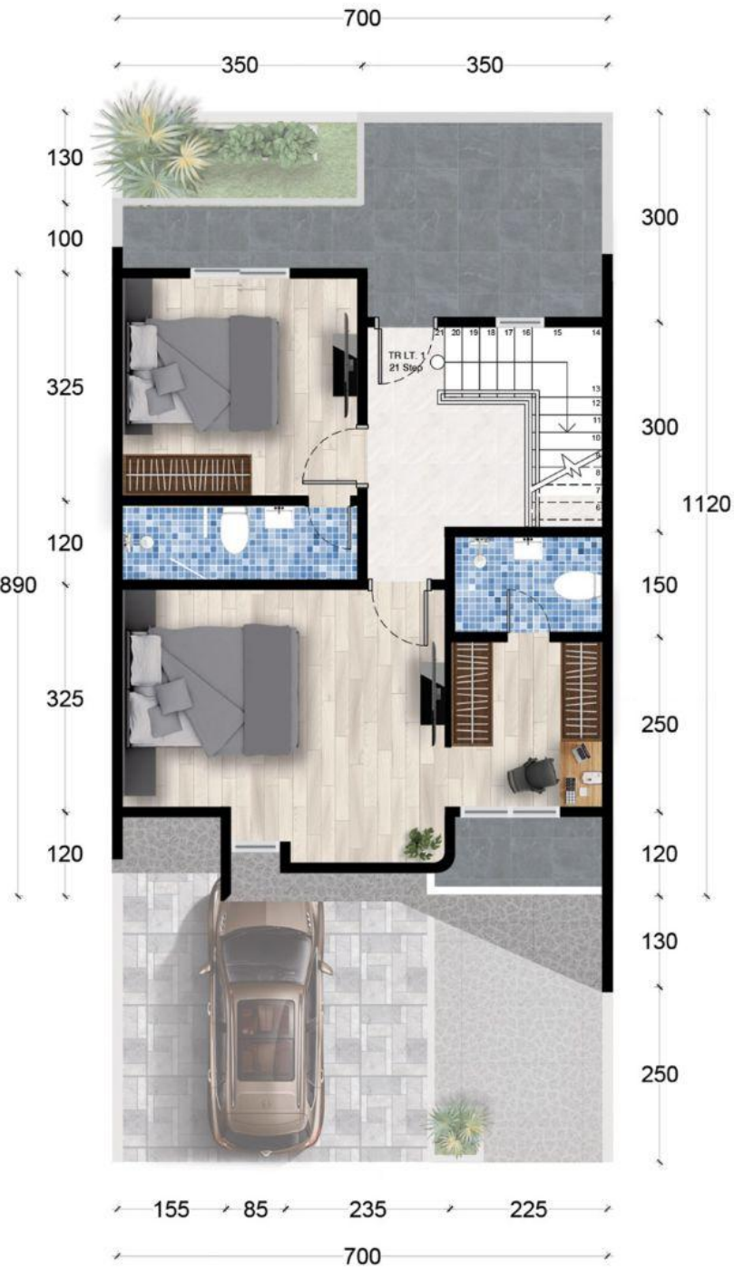
LANTAI 2
