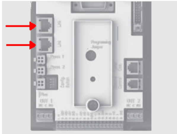
Afbeelding 17: Aansluiting Link
