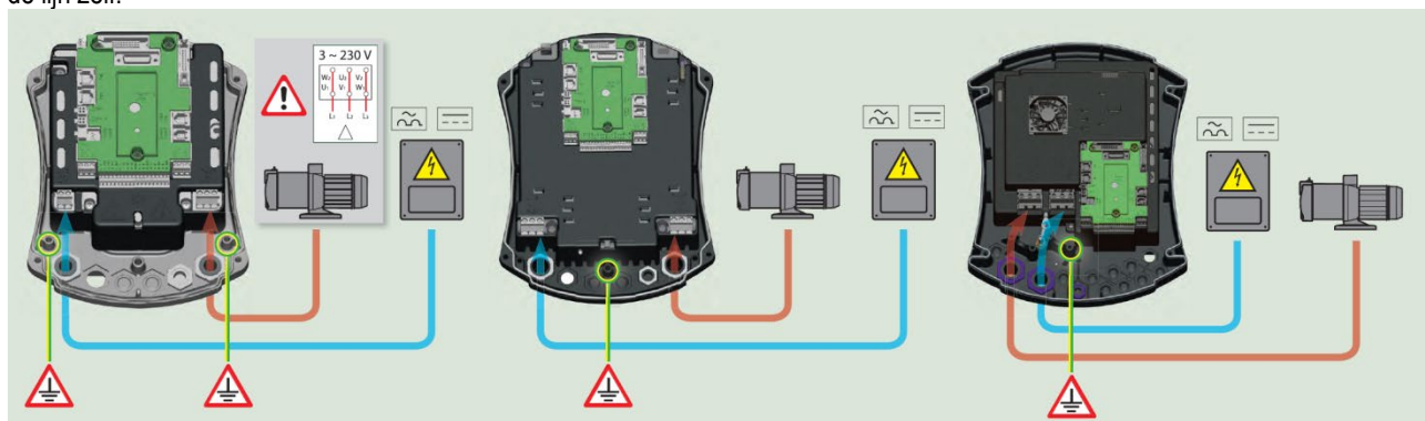
Afbeelding 5: Elektrische aansluitingen
