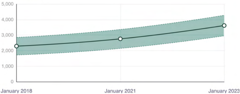
CO2eq. evolution
