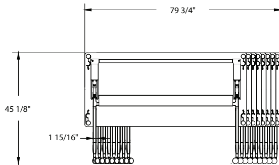
T-Leg nesting
