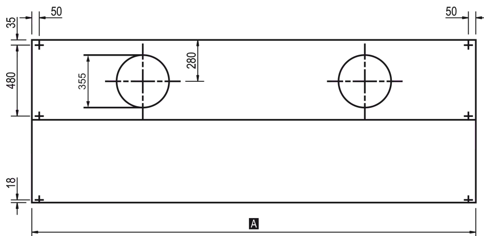
A) Módulo = 1000, 1500, 2000, 2500 ou 3000; Dimensões em mm.
