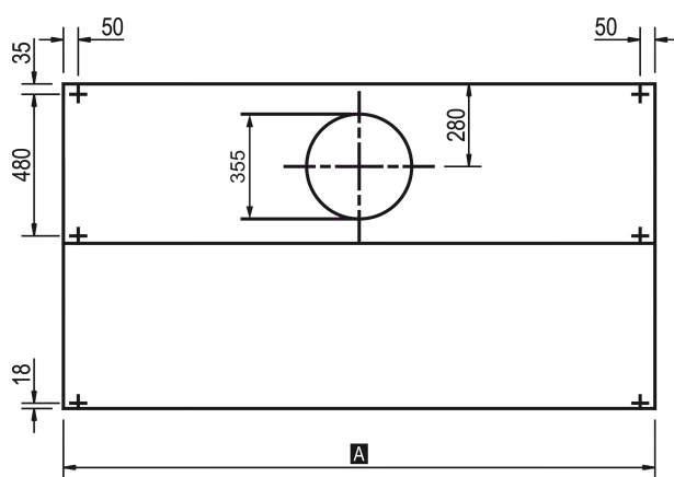
A) Módulo = 1000, 1500 ou 2000; Dimensões em mm.
