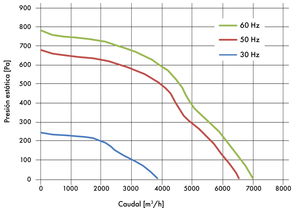
Modelo 500 (MPC F4 T)
