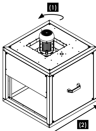
(1) - Motor; (2) - Dirección del aire
