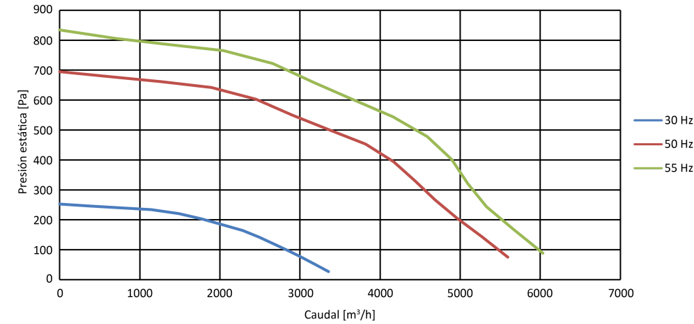
Modelo 450 (MPC F4 TI)
