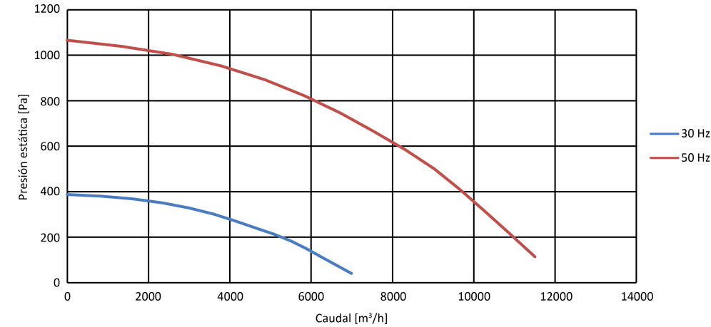
Modelo 560 (MPC F4 TI)
