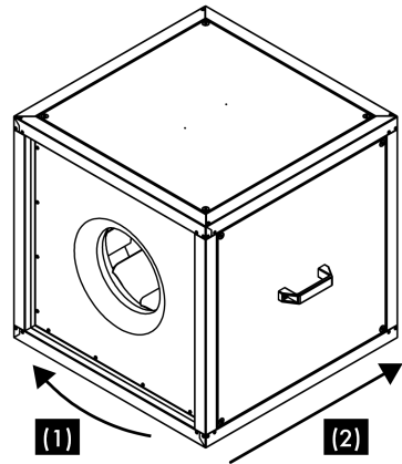
(1) - Motor; (2) - Dirección del aire
