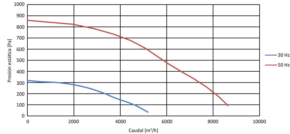
Modelo 500 (MPC F4 TI)
