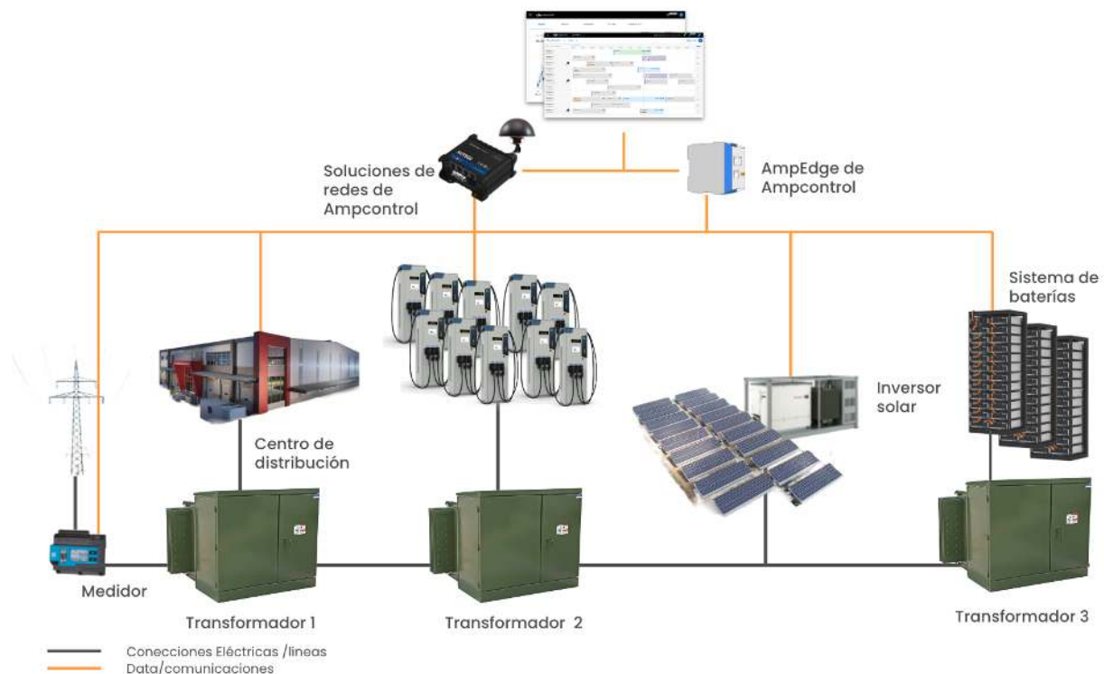
Integración y comunicación de la gestión energética
