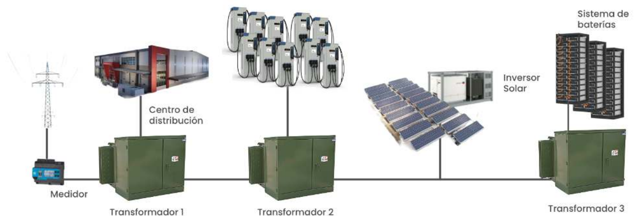
Activos energéticos en el centro de distribución
