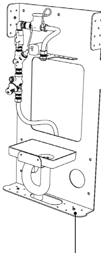
Trägerplatte mit Armatur und Anschlüssen
