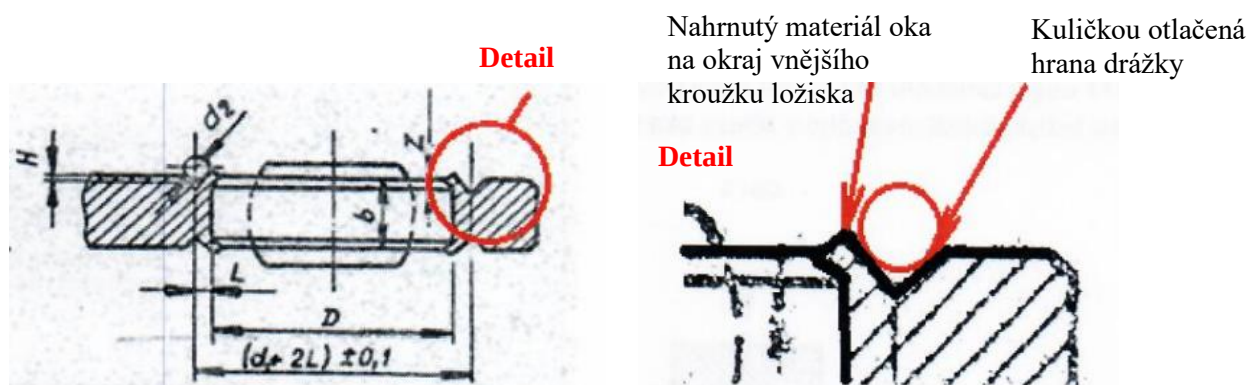
Obr. 3 Správný způsob zajištění ložiska v oku s detailem
