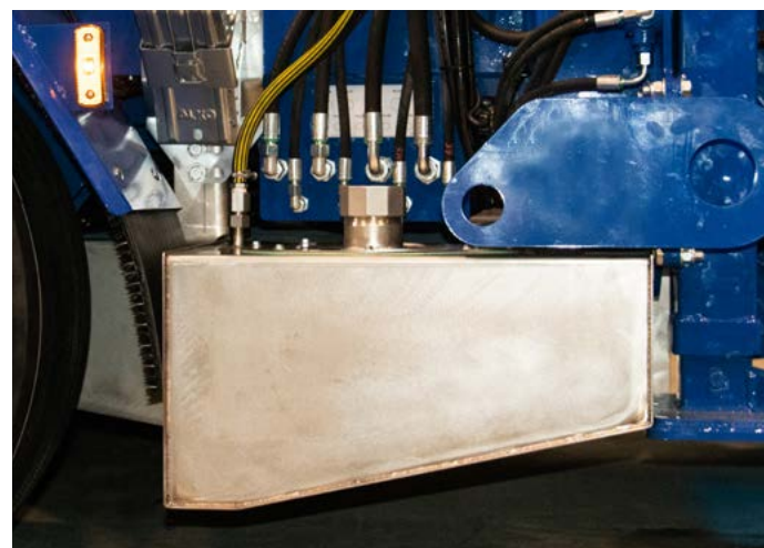
450 l Siliermitteltank
