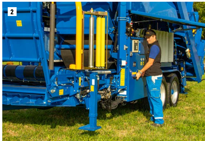
2 Stützfüße ausfahren
