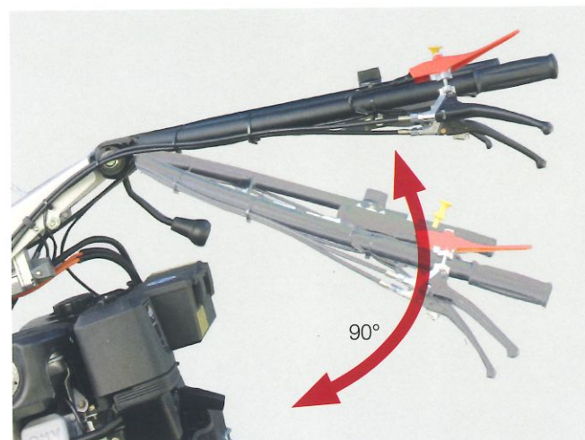
Lenker um 90° abklappbar.
