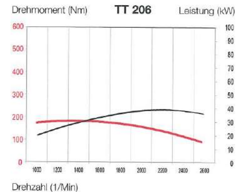
Kubota V2607-CR
