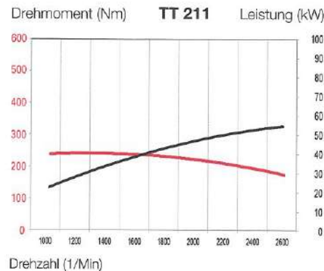
Kubota V2607-CRT/V
