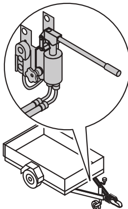
Fig. 54: Elektrisk-hydraulisk pumpe inkl. nødhåndpumpe i almindelig udformning
