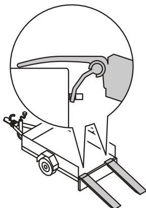
Fig. 40: Påhægtning af sikringskinneren variant B
