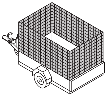
Abb. 37: Gitteraufsatz
