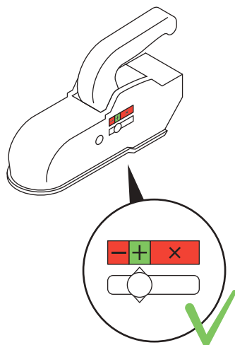
Fig. 6: Koblingens sikkerhets- og slitasjeindikator A1
