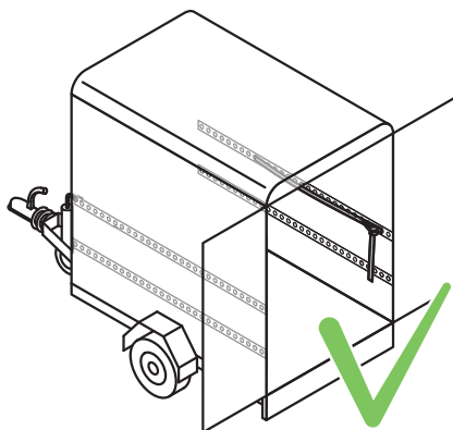
Abb. 31: Richtig verzurrt Ladung
