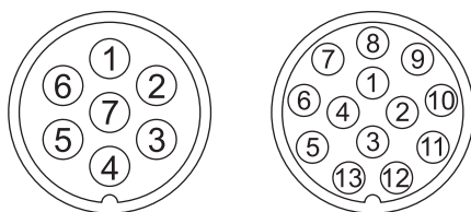
Abb. 1: Ausfertigungen Stecker
