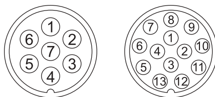
Fig. 1: Utførelser plugg
