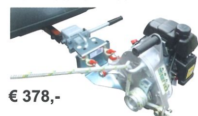
Schnellverschluss für Anhängerkugel PCA1266/PCA1268
