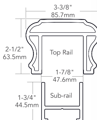
Horizontal Baluster
