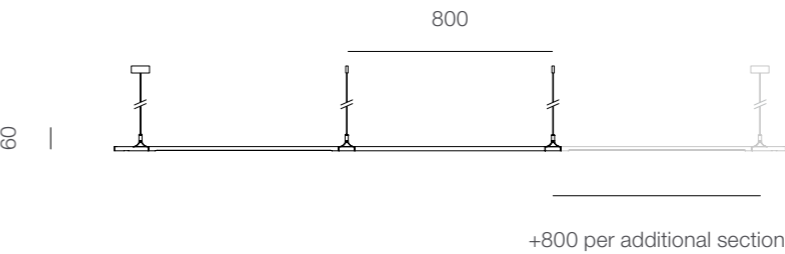
PENDANT 3, 4, 5 SECTIONS
