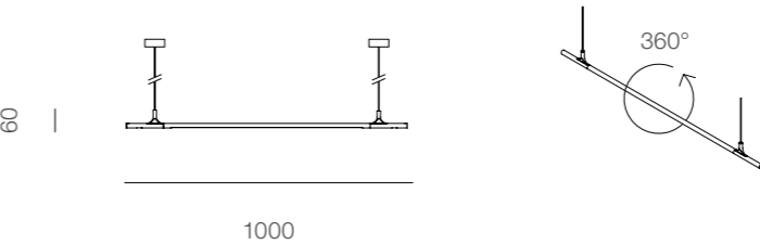
PENDANT 2 SECTIONS
