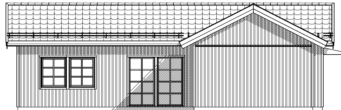
FASAD 4
