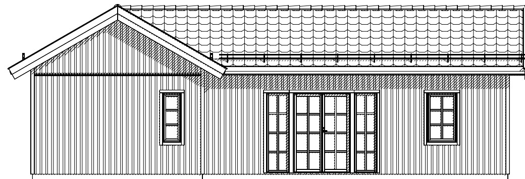
FASAD 3
