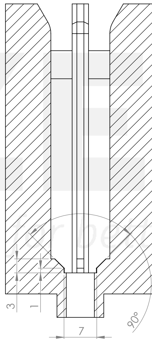
A-A (2 : 1)
