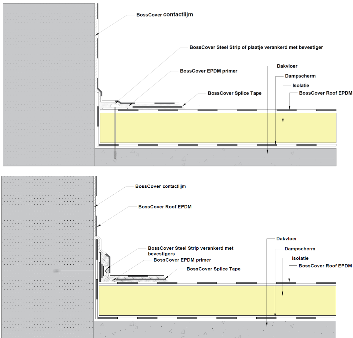
Fig. 8 – Kimfixatie met aparte strook (alternatieve kimfixatie) – horizontale bevestiging in dakvloer en verticale bevestiging in opkant
