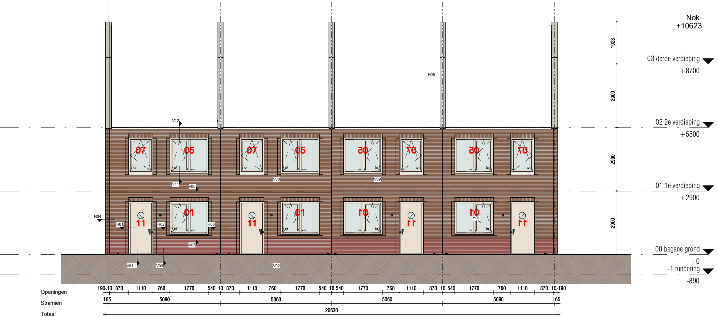
Voorgevel
