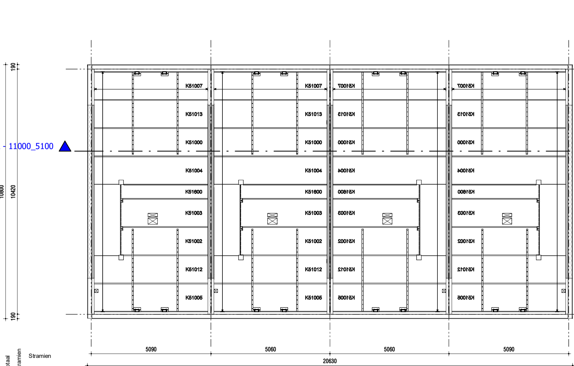
2e verdieping
