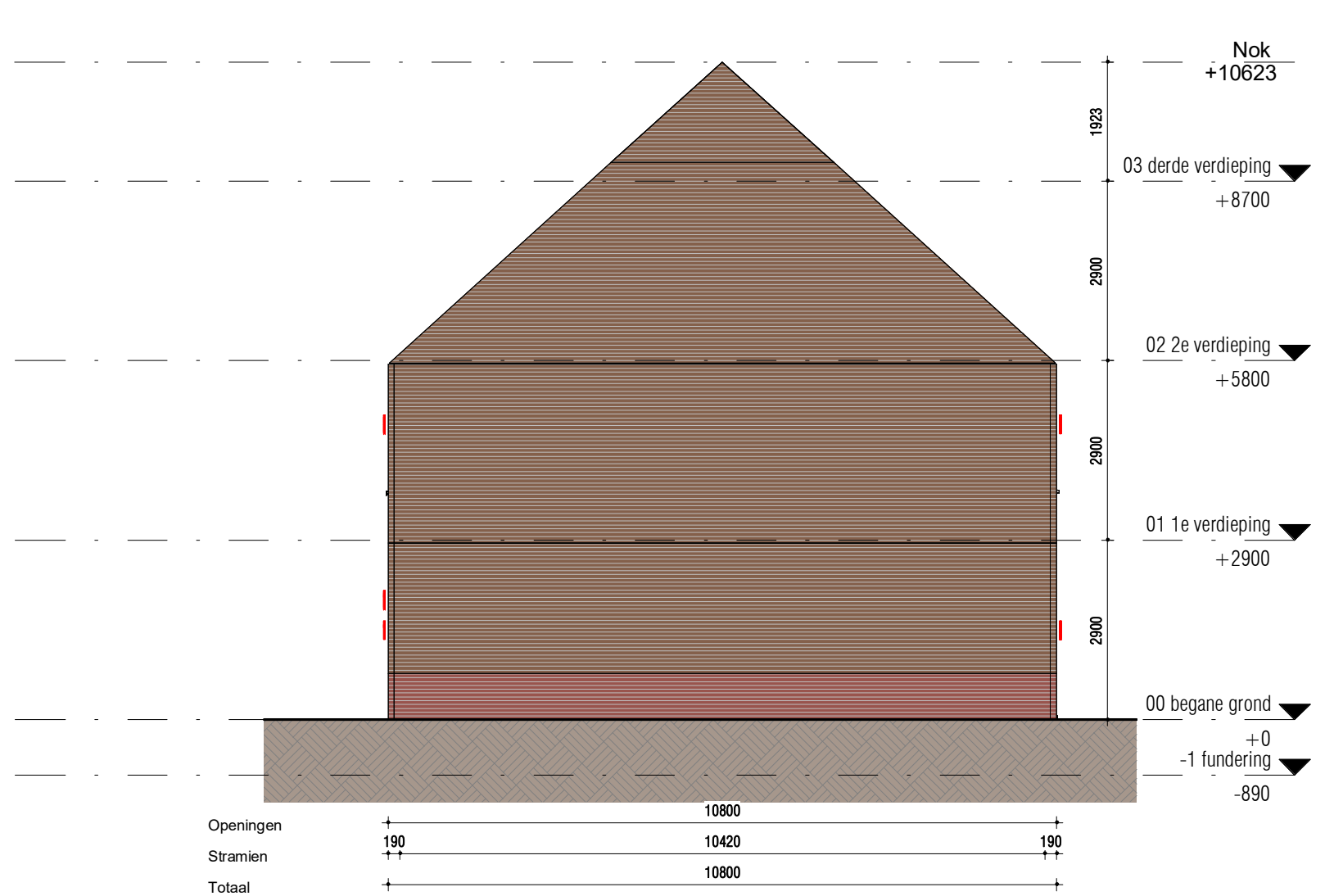
Rechtergevel
