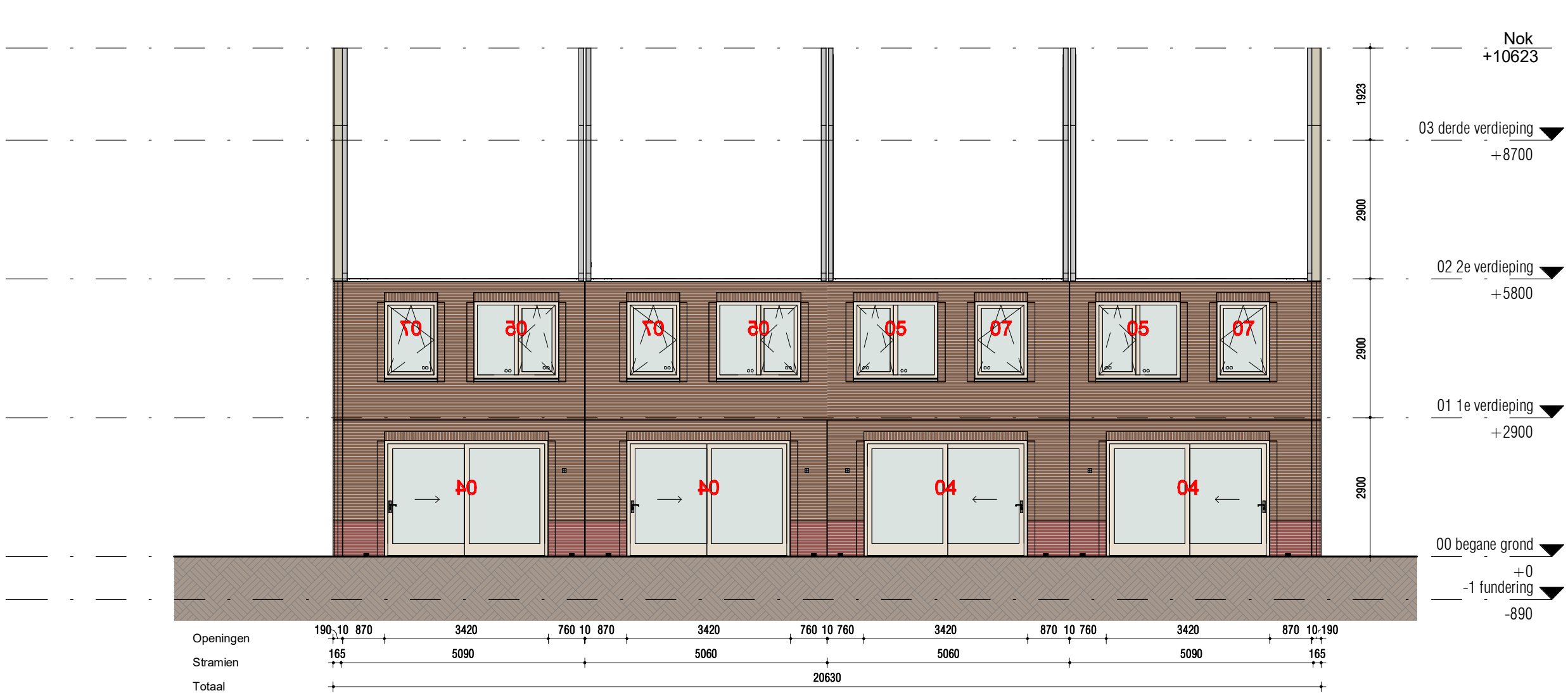
Achtergevel
