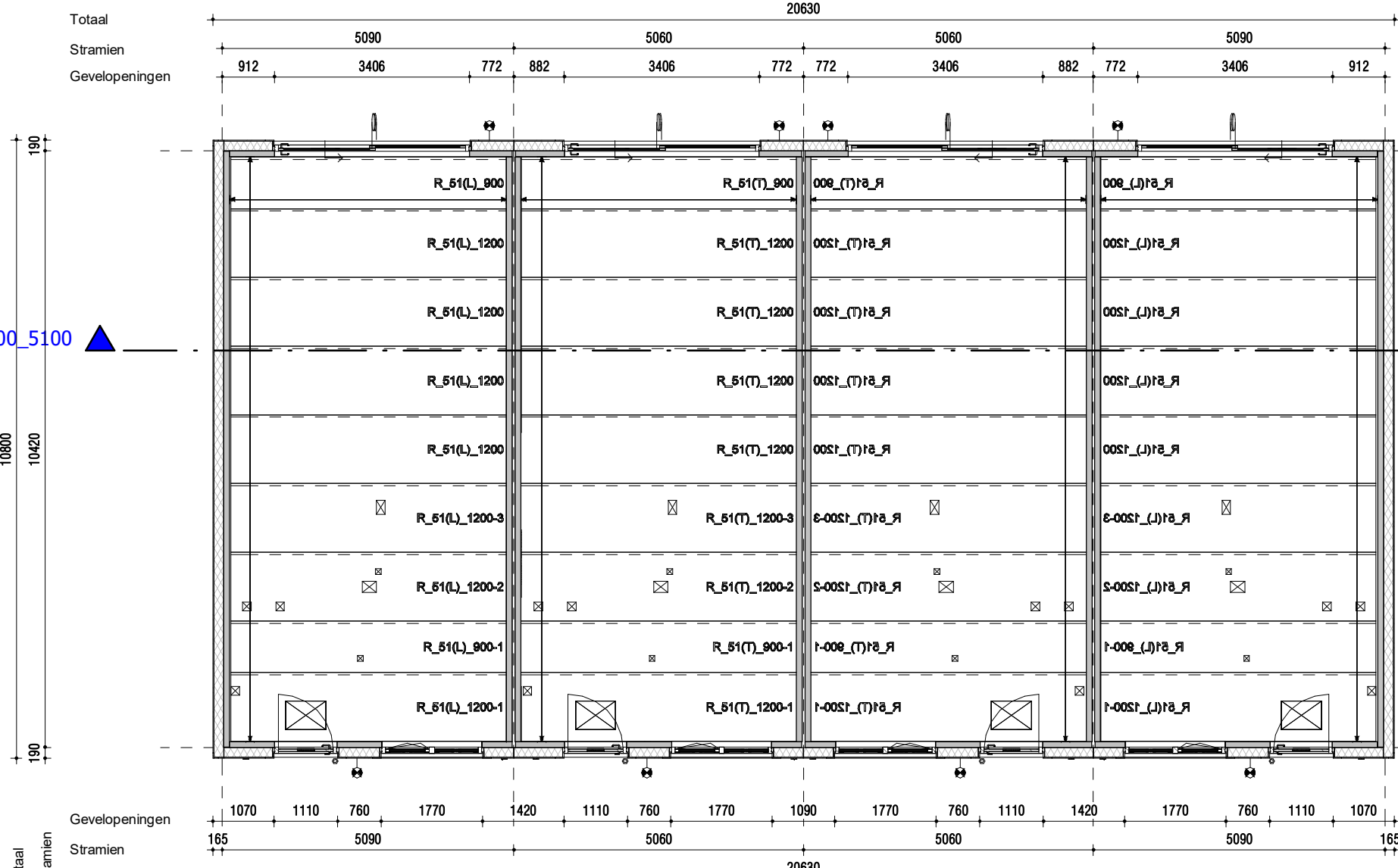
begane grond
