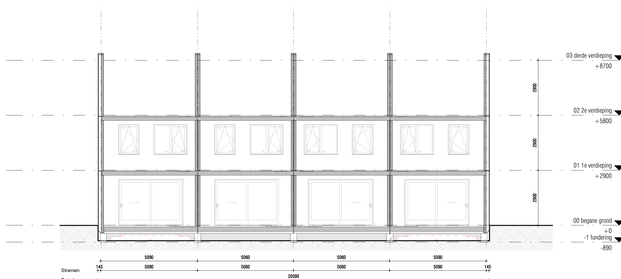
Doorsnede A-A
