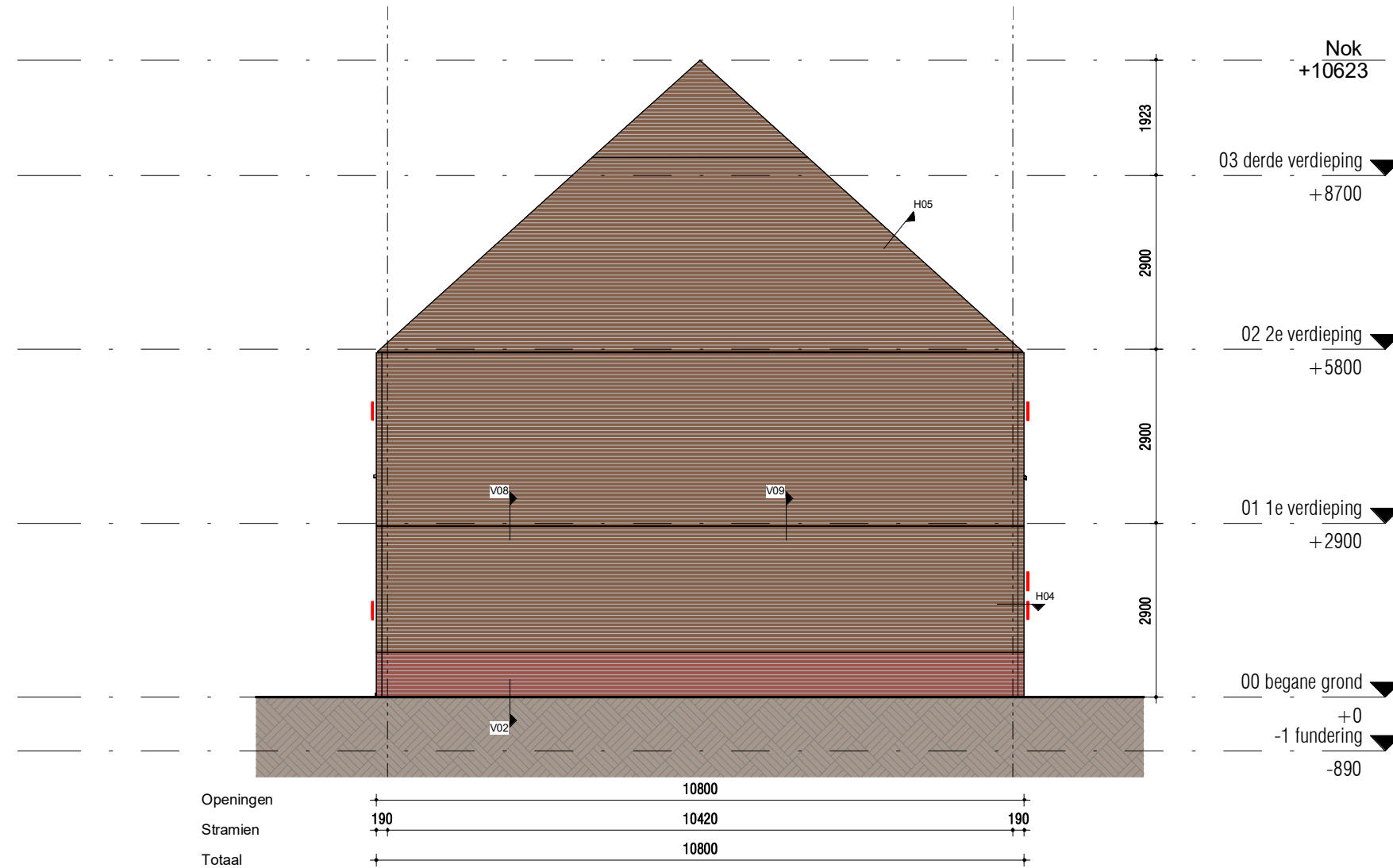
Linkergevel
