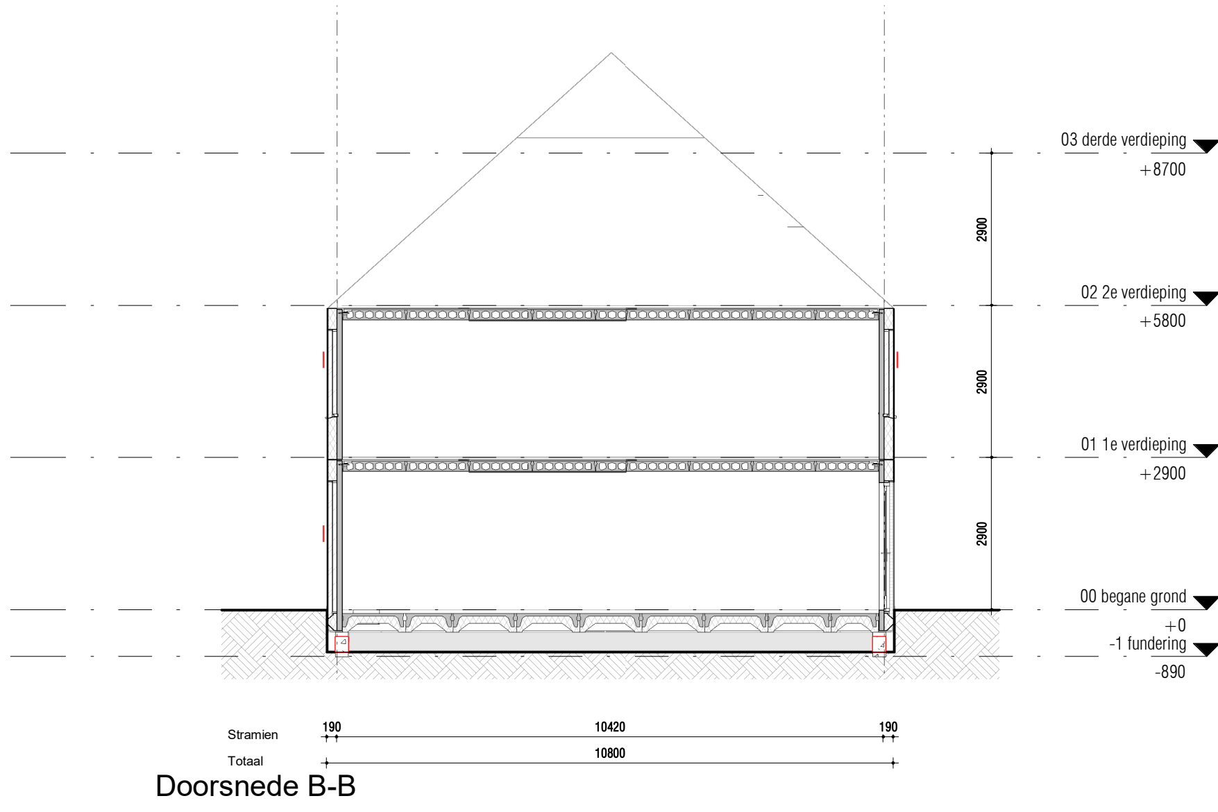
Doorsnede B-B
