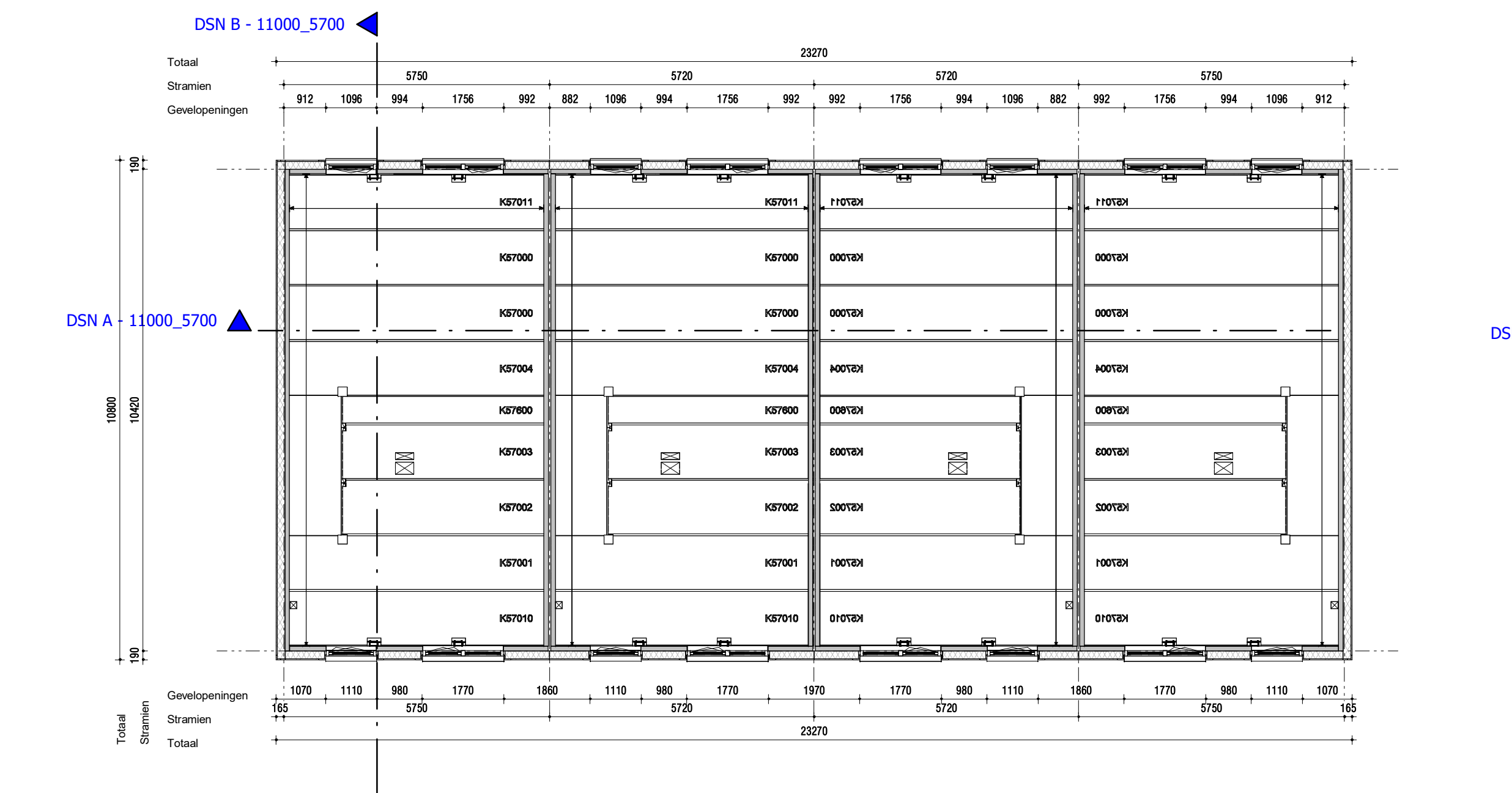
1e verdieping
