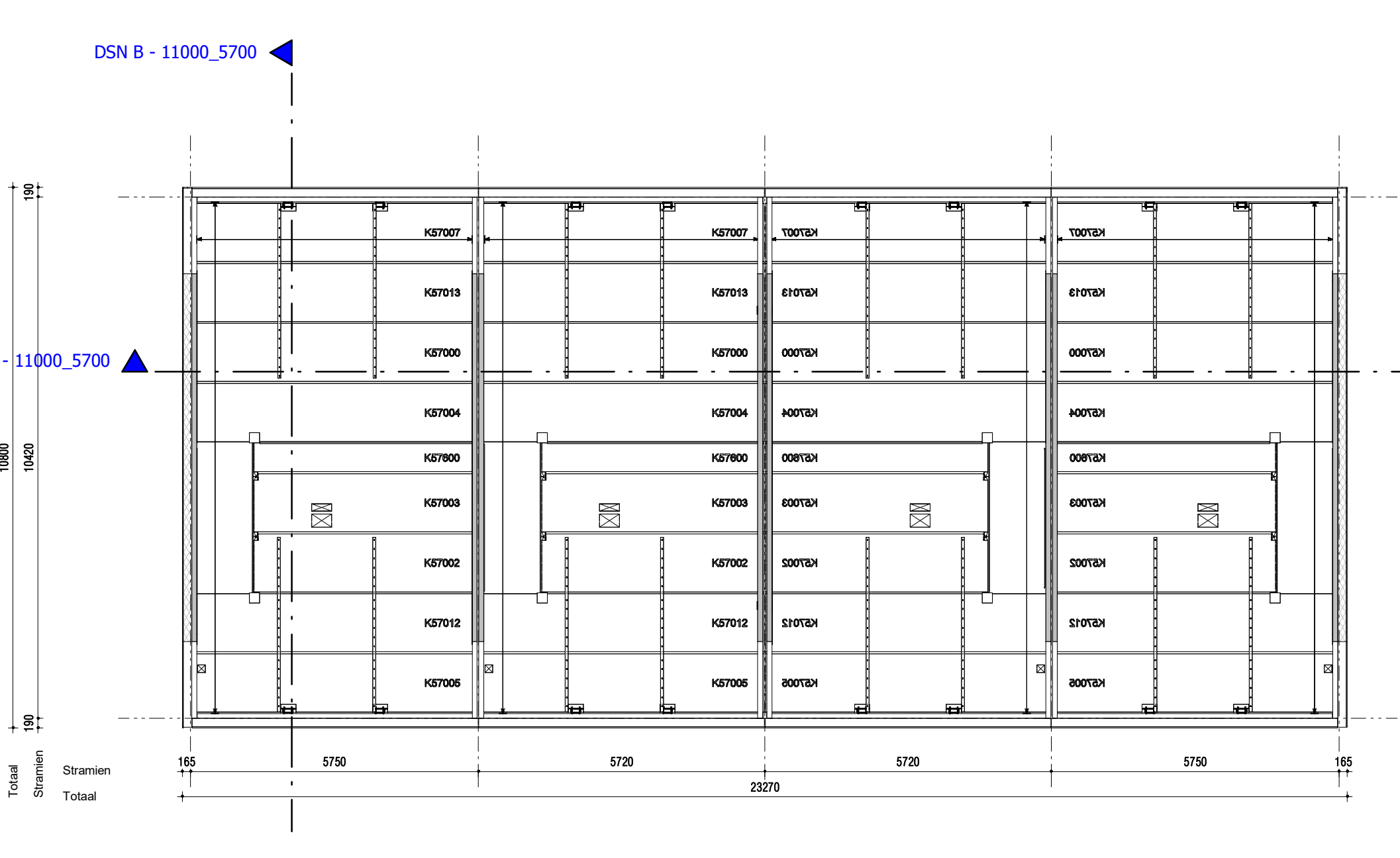
2e verdieping
