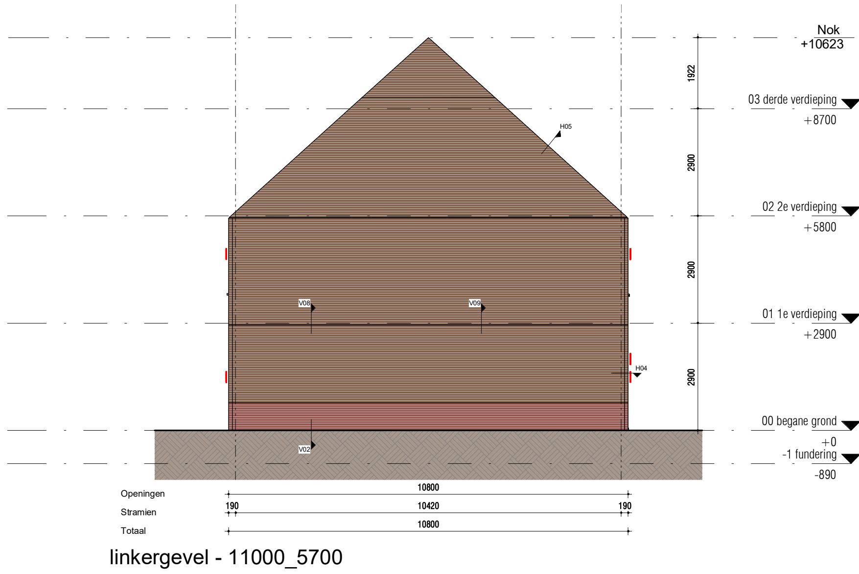
linkergevel - 11000_5700
