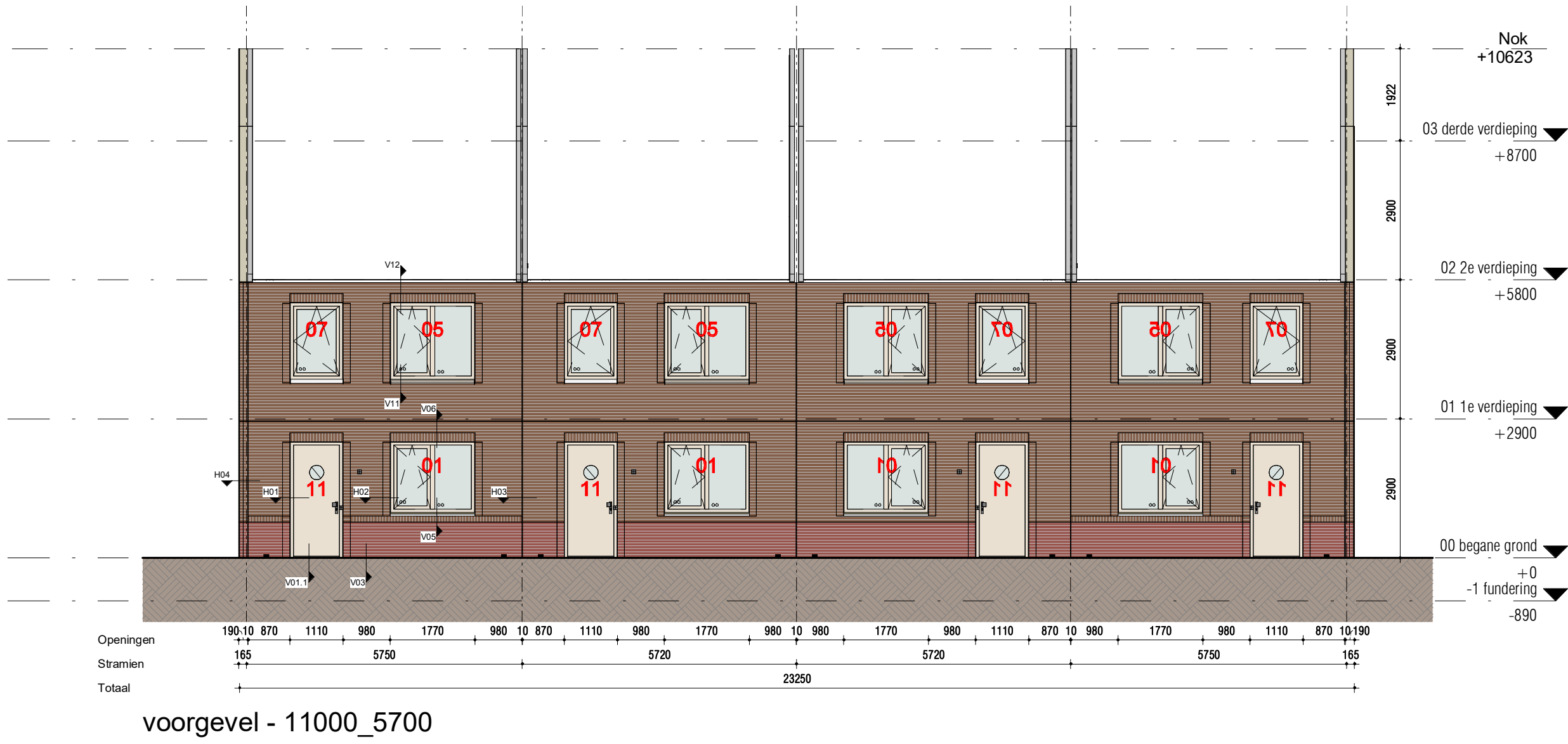
voorgevel - 11000_5700
