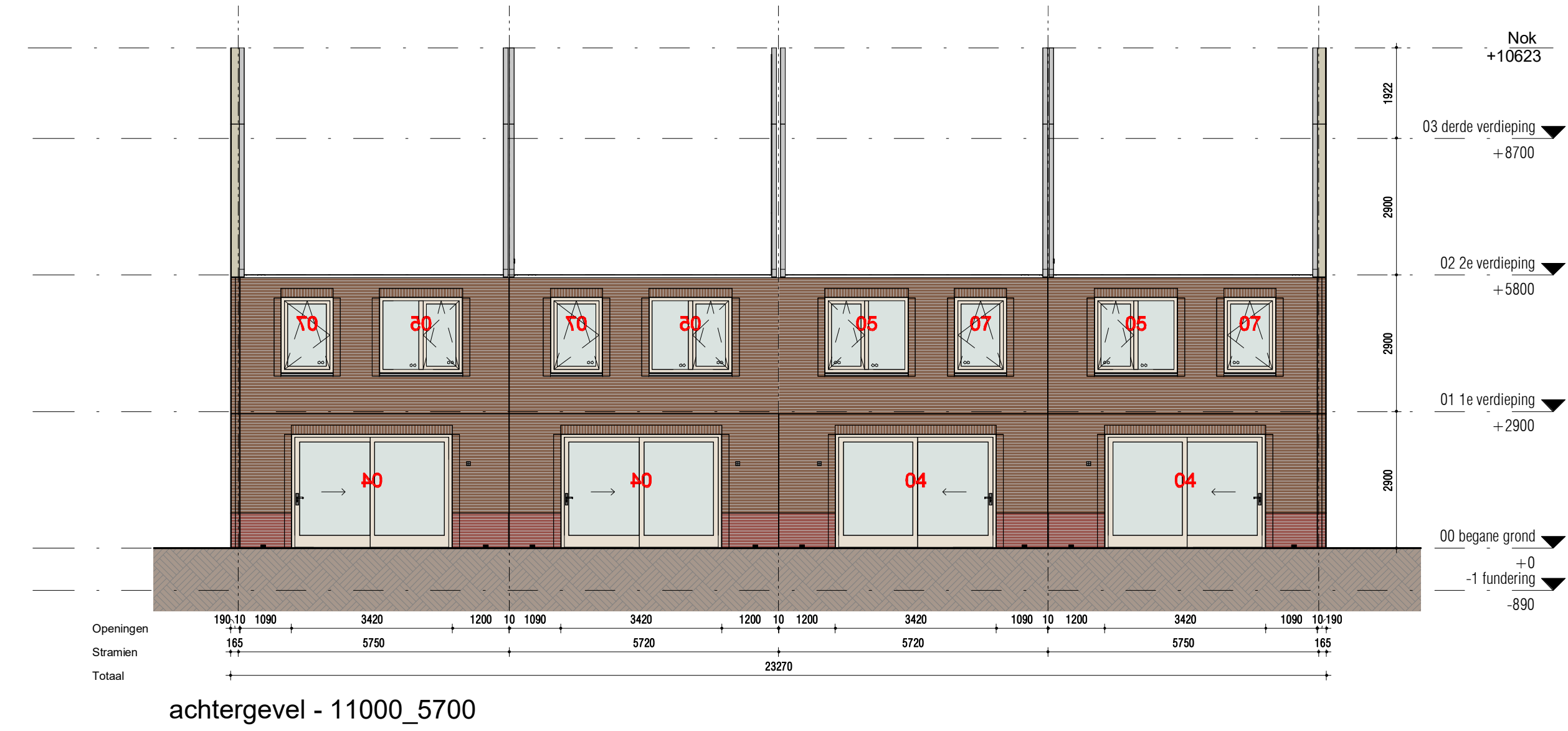
achtergevel - 11000_5700
