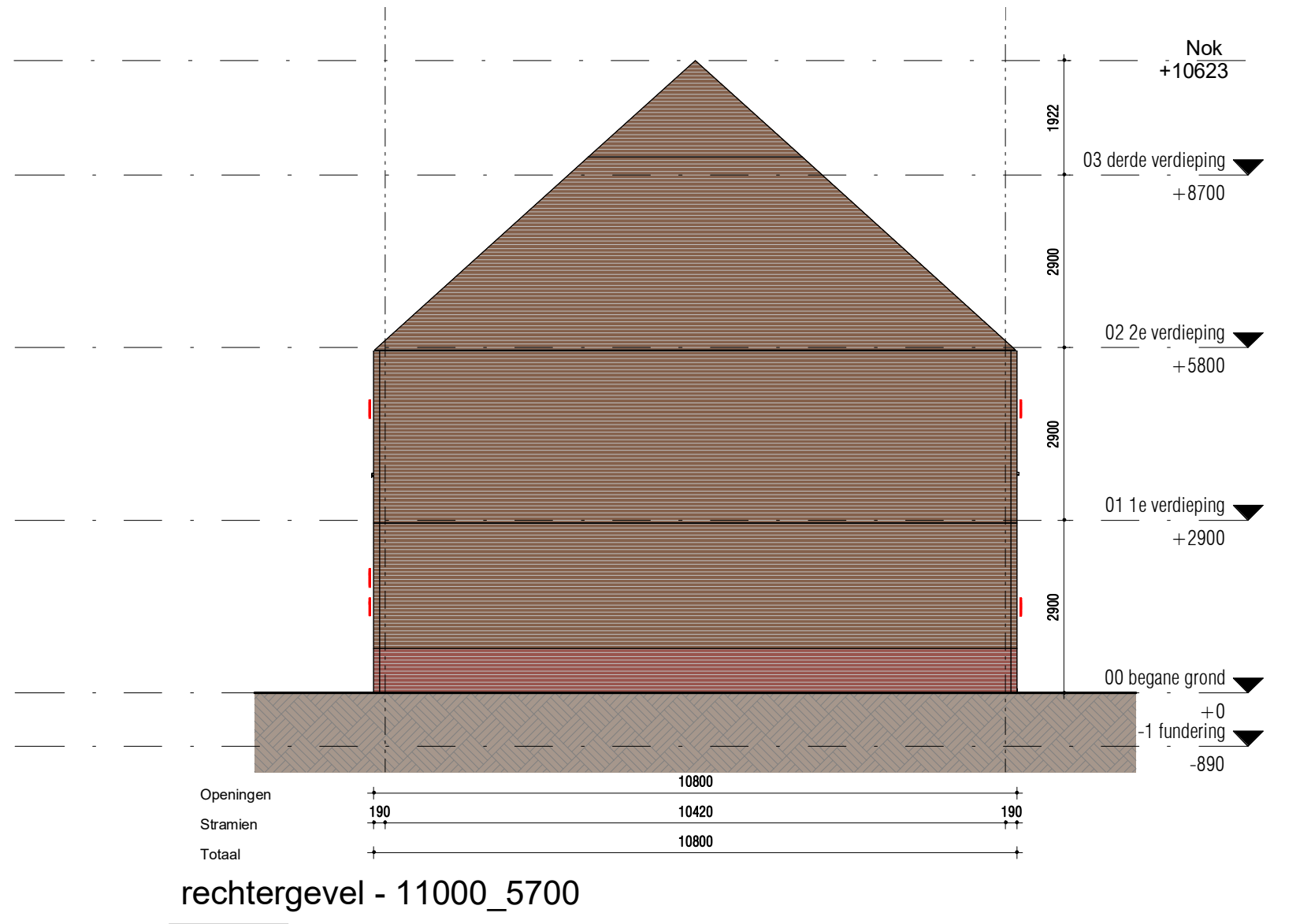
rechtergevel - 11000_5700
