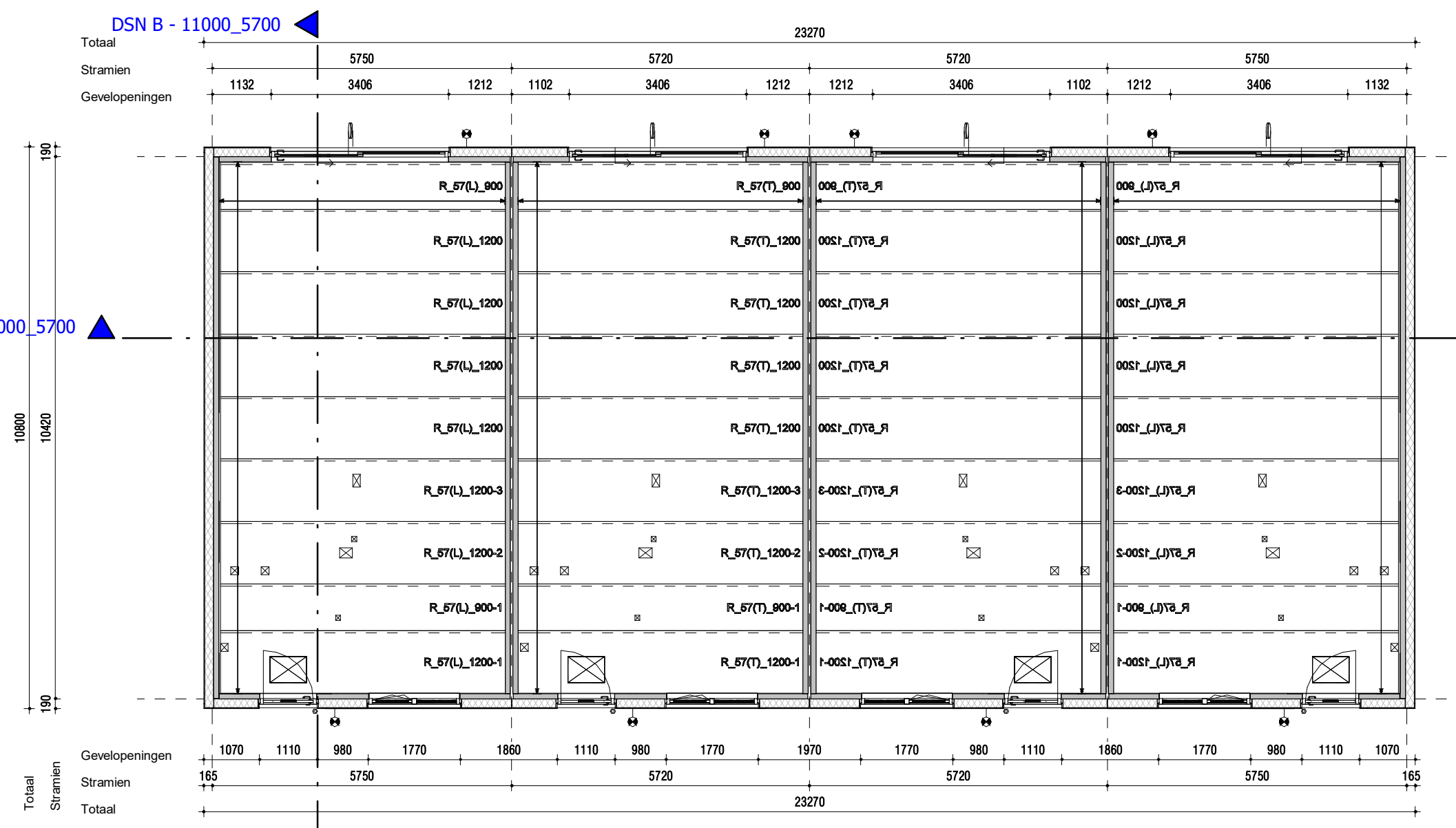
begane grond
