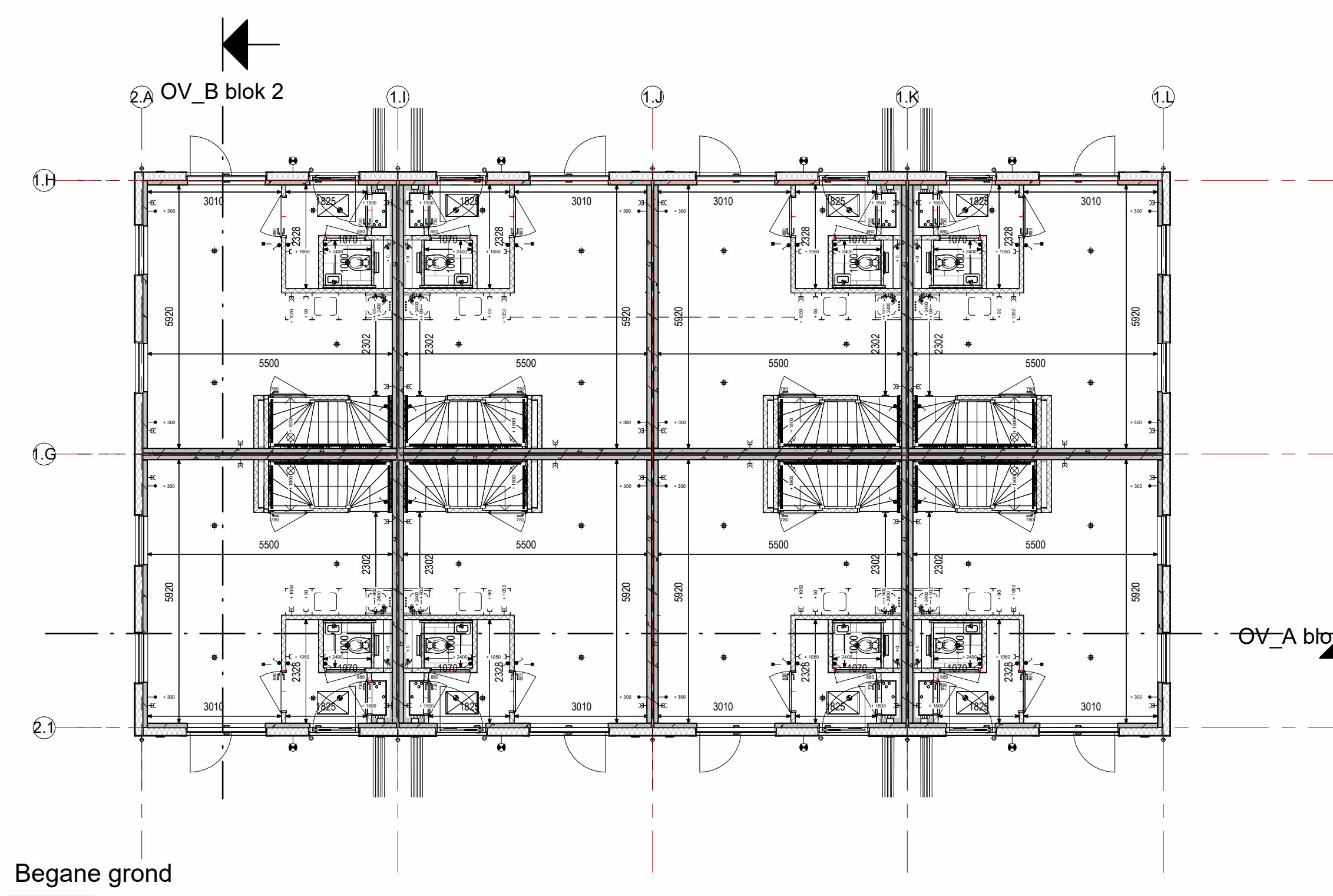
Begane grond
