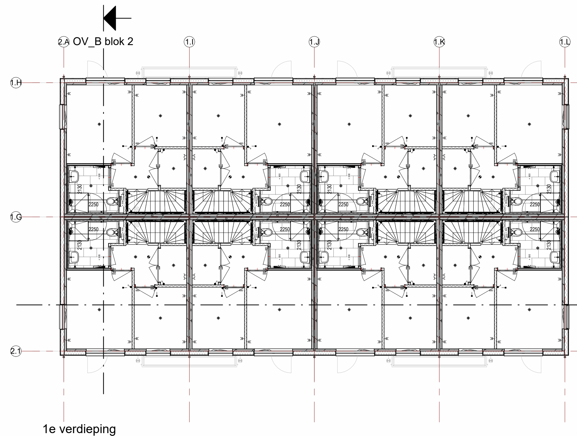
1e verdieping
