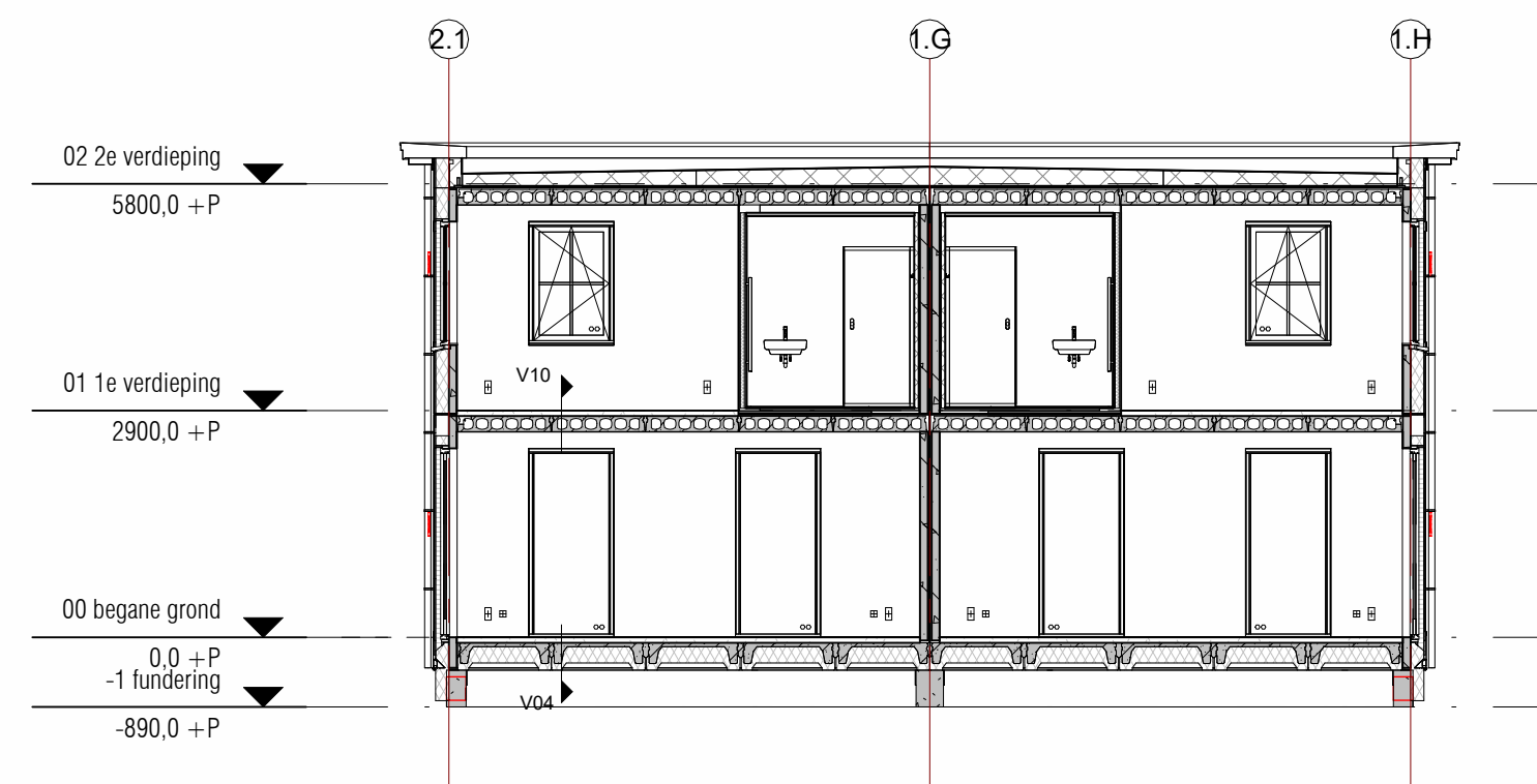
Doorsnede D-D
