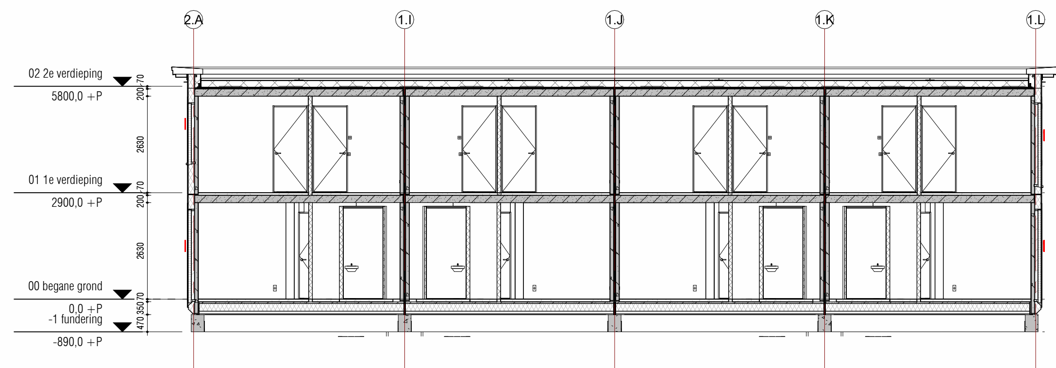
Doorsnede C-C
