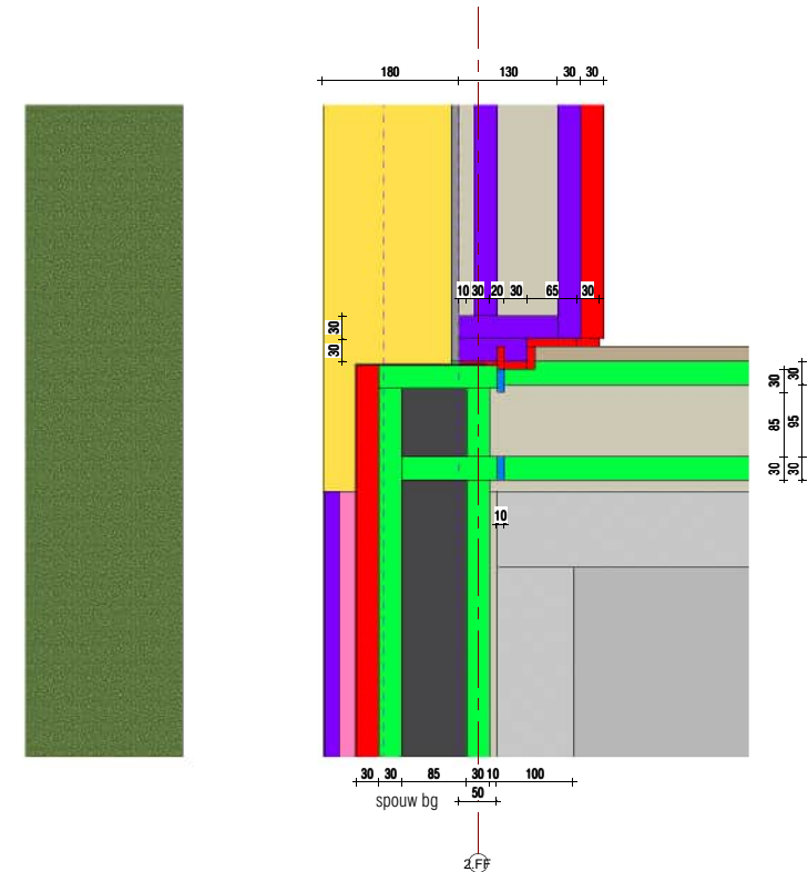
22 dilatatie achtergevel - spouw 50mm
