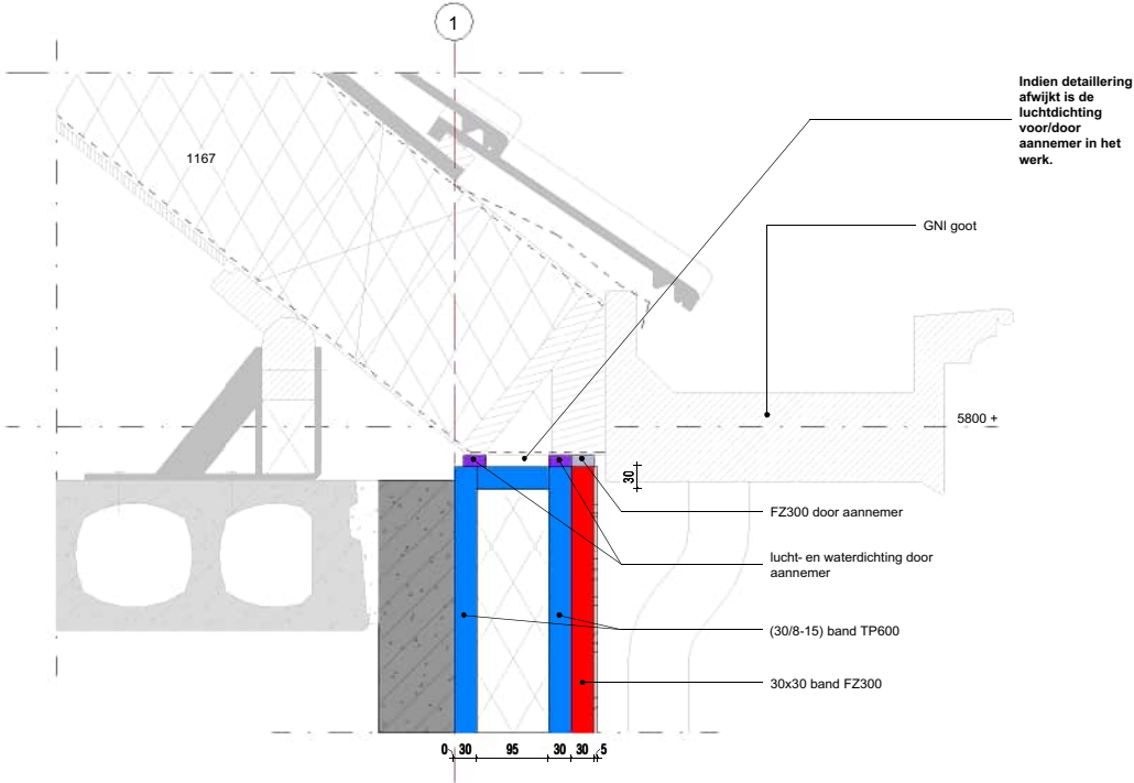
11 boven aansluiting kozijn met dak, basis kozijn GNI goot
