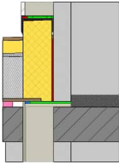
Verticale doorsnede
