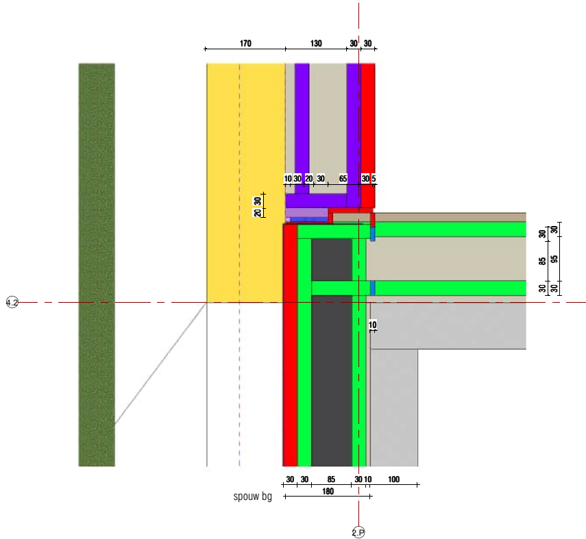
22 dilatatie achtergevel - spouw 180mm
