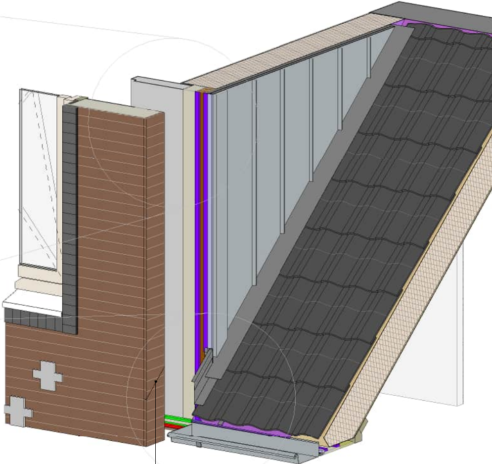
loodslabbe door aannemer in het werk aanbrengen
