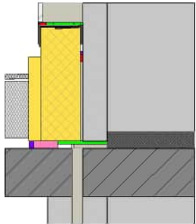
Verticale doorsnede
