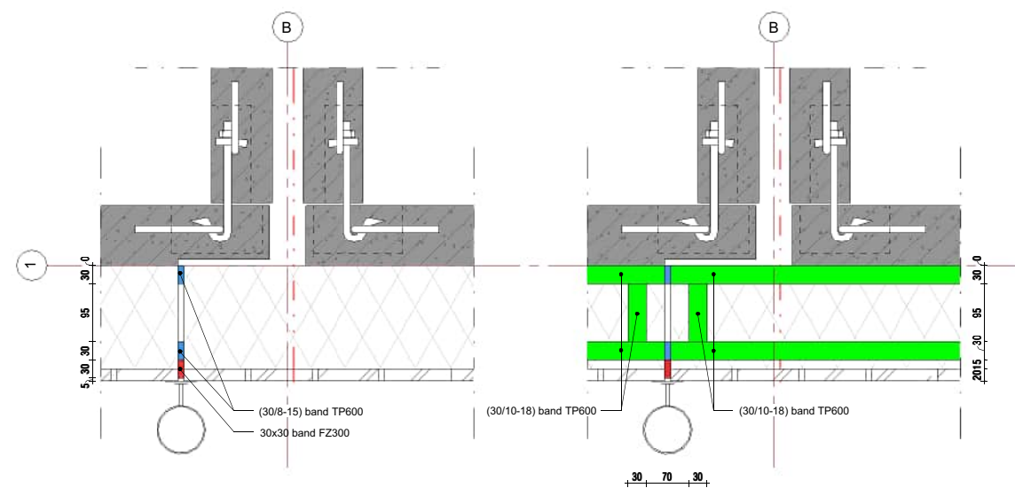
06B aansluiting scheiding wand
