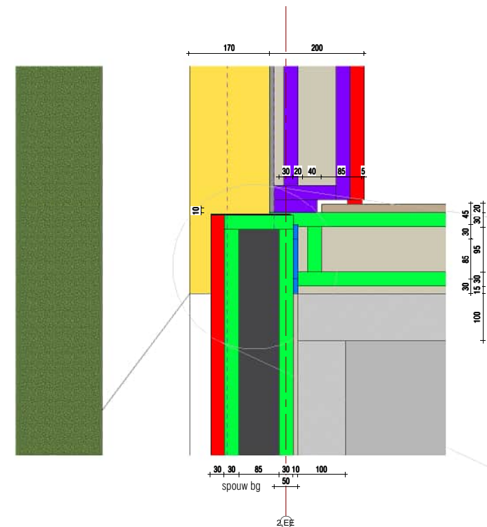
21 dilatatie zijgevel - spouw 50mm
