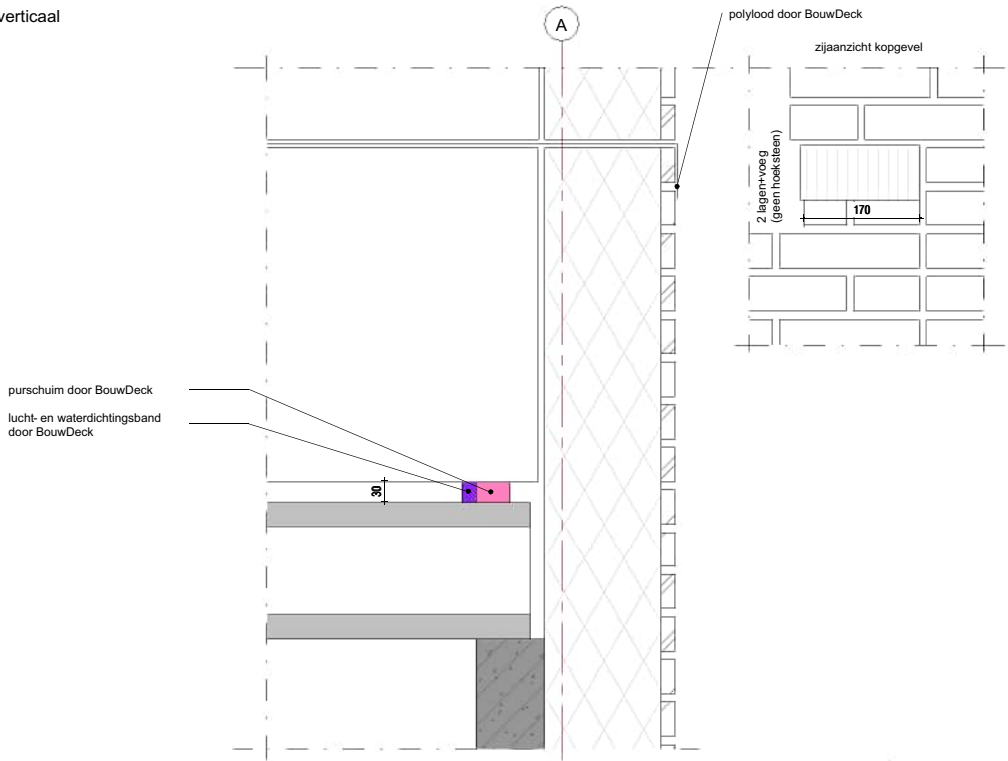
03A3.2 uitbouw verticaal
