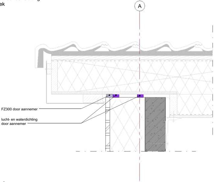
12 dak met muur aansluiting met overstek
