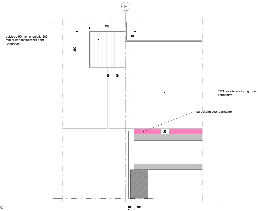
03A3.1 aansluiting luifel voorgevel
