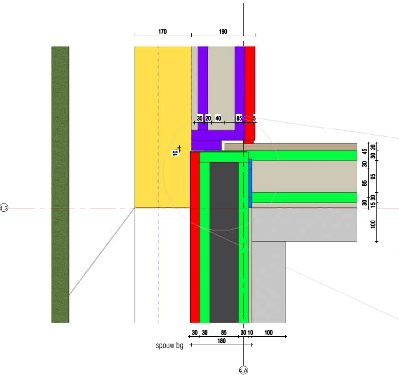
21 dilatatie zijgevel - spouw 180mm
