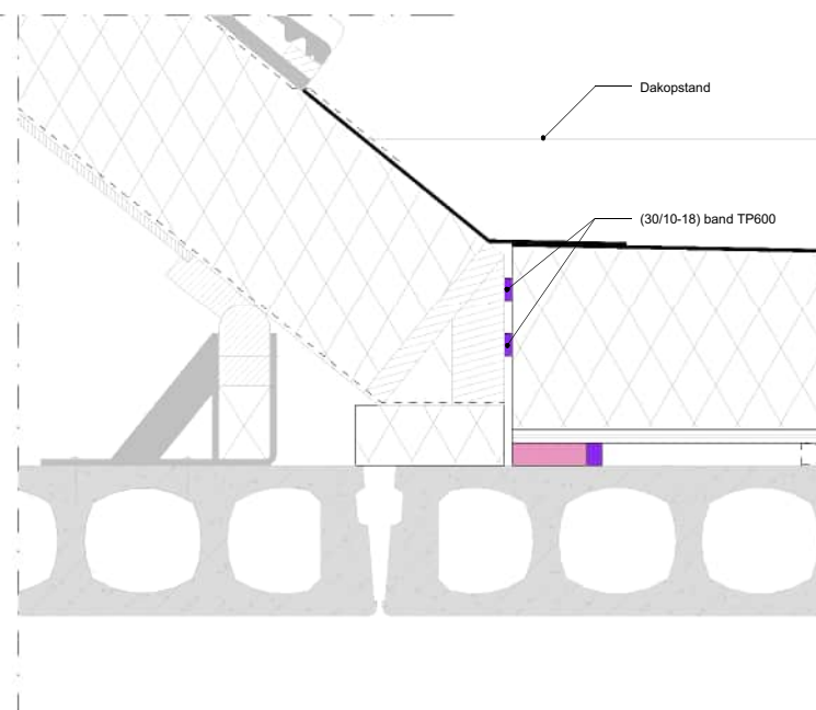
29 aansluiting Bouwdeck met dakkap
