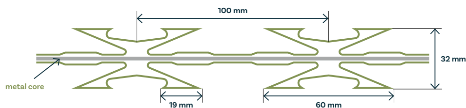
CBT 60 dimensions
