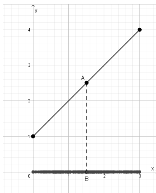
Figura 2. Rastro de un punto de la gráfica de f proyectado sobre el eje X .
