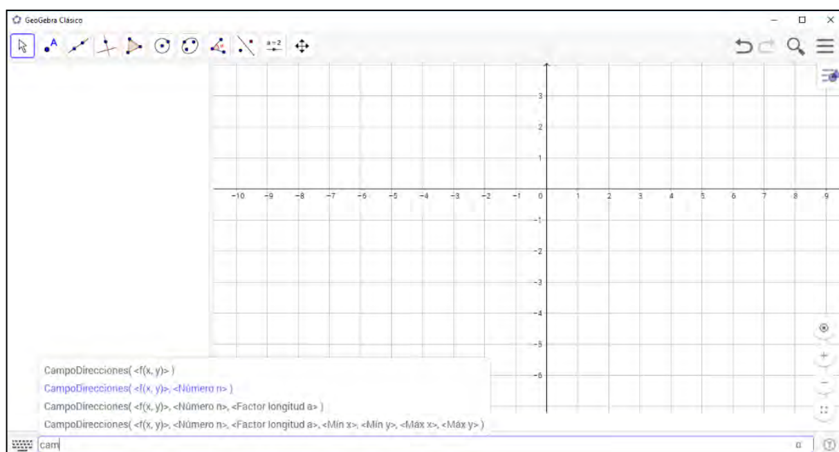
Figura 1. Inicio de construcción de Campo de Direcciones
