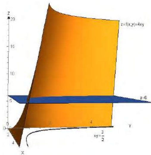
Figura 3. Curva de nivel de f correspondiente a c = 6 .
