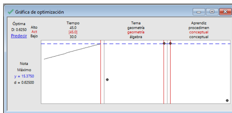
Figura 8. Gráfica de maximización para variable. Nota con interacción de tres factores.
