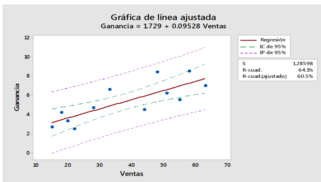
Figura 5. Gráfica de línea de regresión y de intervalos de confianza y predicción, para ventas vs ganancia.
