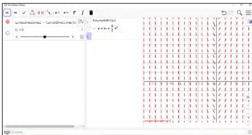
Figura 7. Gráfica del campo de direcciones de \frac{dy}{dx} = 5x
