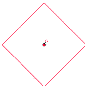
Figura 1. Circunferencia \mathcal{C}_T .
