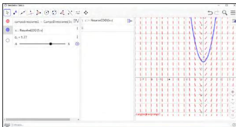
Figura 8. Gráfica del campo de direcciones y solución de \frac{dy}{dx} = 5x
