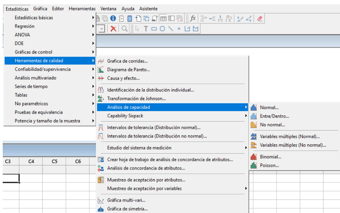
Figura 1. Ventana de trabajo y opciones del software Minitab para el estudio de la calidad.
