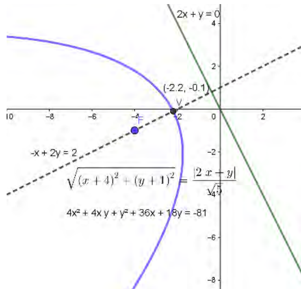
Figura 3, Parábola \mathcal{P}_E
