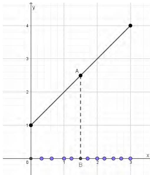
Figura 1. Proyección ortogonal de un punto de la gráfica de f sobre el eje X .
