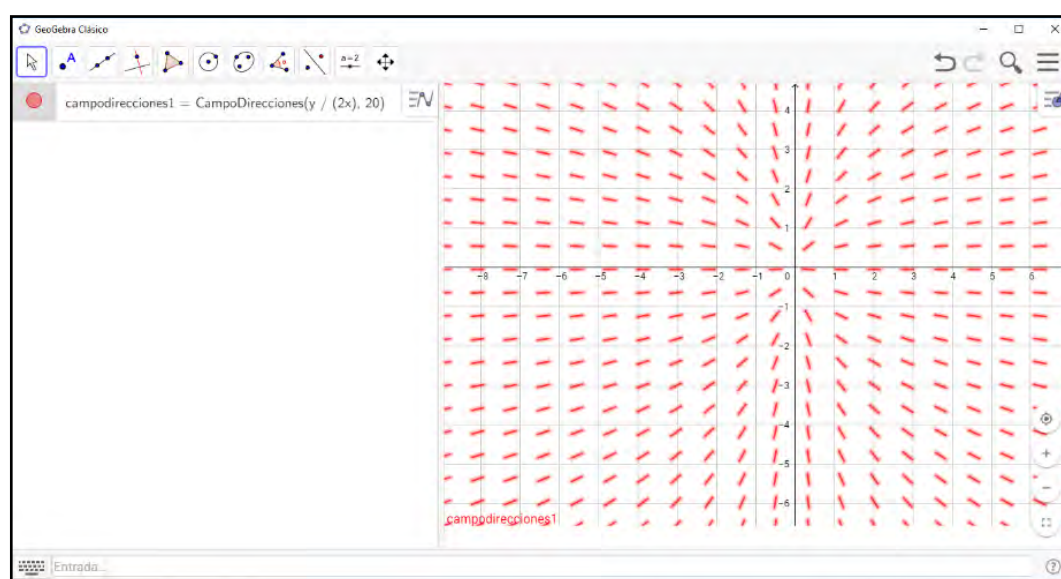
Figura 3. Campo de direcciones de \frac{dy}{dx} = \frac{y}{2x} .
