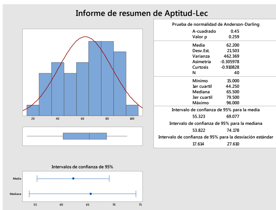
Figura 4. Principales estadísticos y gráfica de histograma para la variable aptitud lectora.
