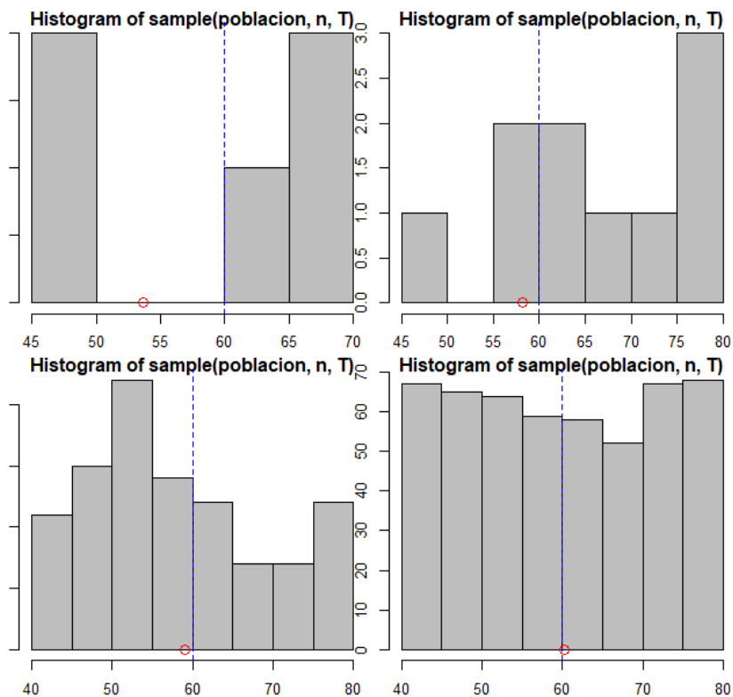
Figura 4. Distribución de una muestra de tamaño 5, 10, 100 y 500, y representación del valor del estimador respecto al parámetro de 60.
