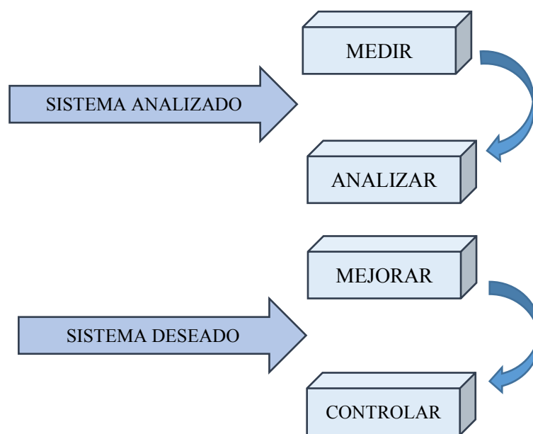
Figura 3. Fases operativas (para el trabajo con datos) de un proyecto 6 \sigma .
