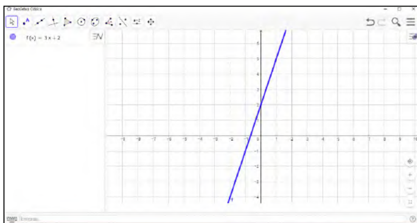
Figura 1. Trazo de la recta y = 3x + 2 .
